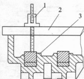
图 4.1.3-1 缓冲器相对标高测量
