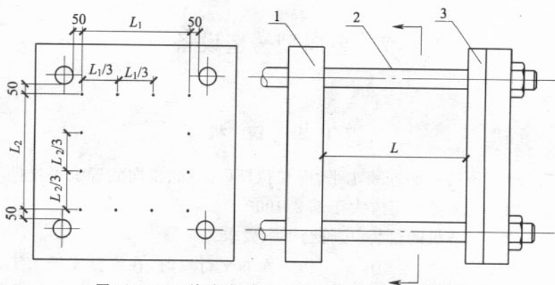
图 7.1.2-1 检验动、定型座板工作表面间的平行度
