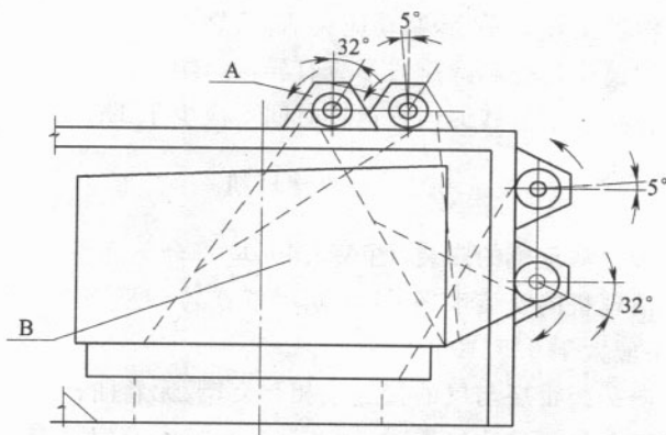
图 6.1.1 抛丸矩形窗口的安装位置 A—定向套;B—被清理件放置区域
