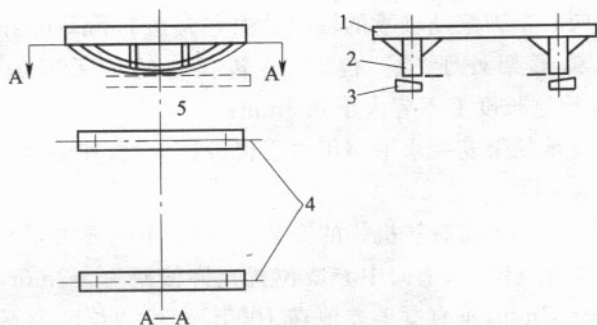
图 9.3.2 弧形架安装
