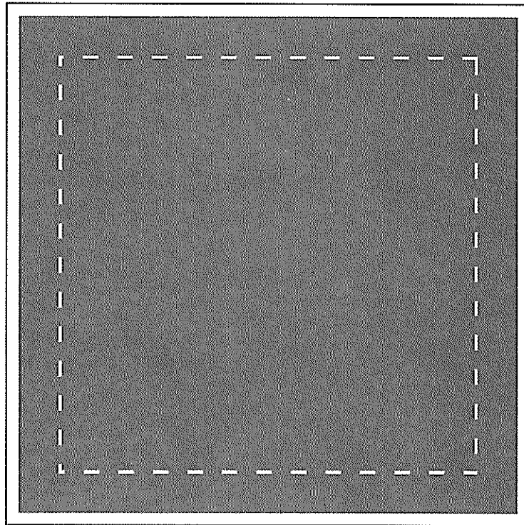
图 11 安全条件标志的符号设计模板
