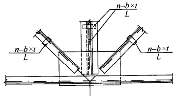
图 4.4.6 缀板的标注方法
