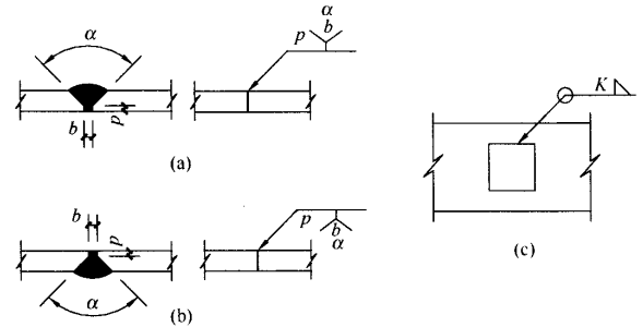
图 4.3.2 单面焊缝的标注方法
