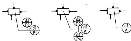
(a)同方向节点相同 (b)d1与d3相同,d2与d4不同 (c)所有节点相同
