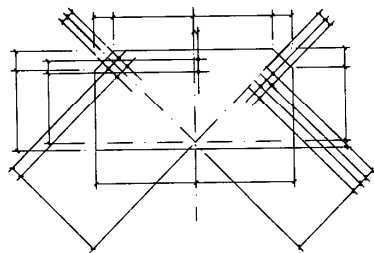
图 4.4.7 非焊接节点板尺寸的标注方法
