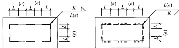
图 4.3.7 不规则焊缝的标注方法
