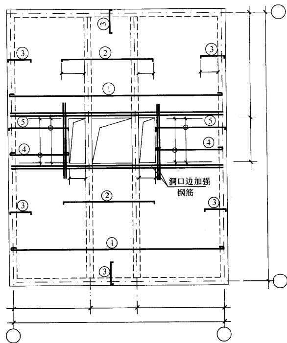
图 3.1.4-2 楼板配筋较复杂的表示方法
