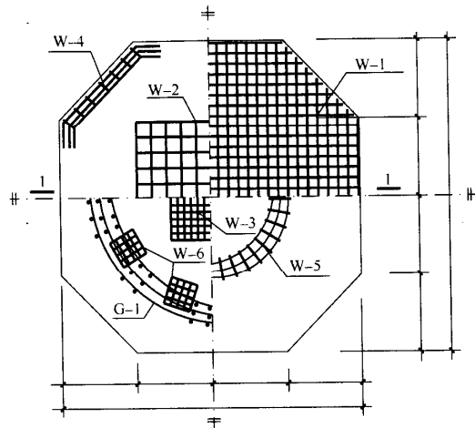
图 3.2.1 构件中钢筋简化表示方法
