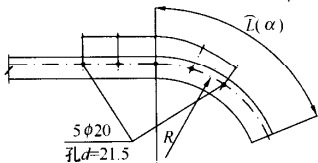
图 4.4.2 弯曲构件尺寸的标注方法
