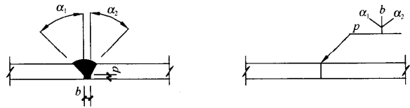
图 4.3.6 不对称坡口焊缝的标注方法
