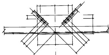
图 4.4.5 节点尺寸的标注方法
