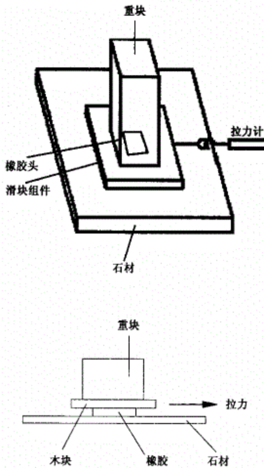
图 1 防滑系数测试示意图
