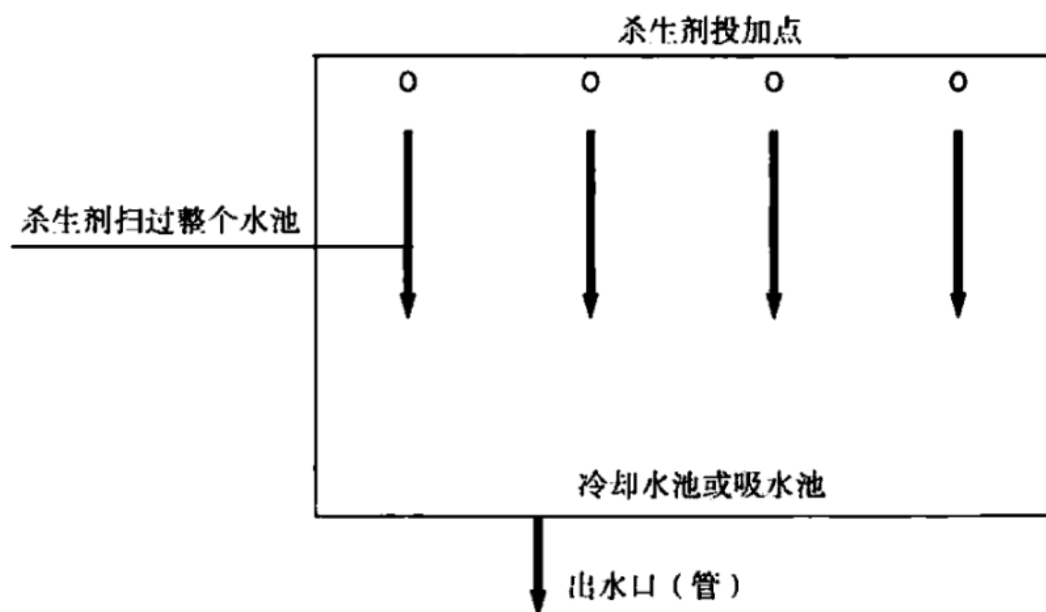
图1 杀生剂的投加点位置
