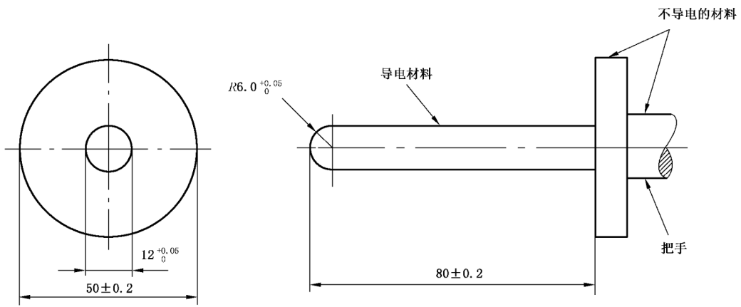
图 A.3 钝头试具
