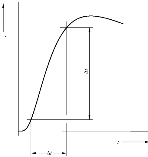
图 C.2 根据表 C.3 定义的雷电流陡度
