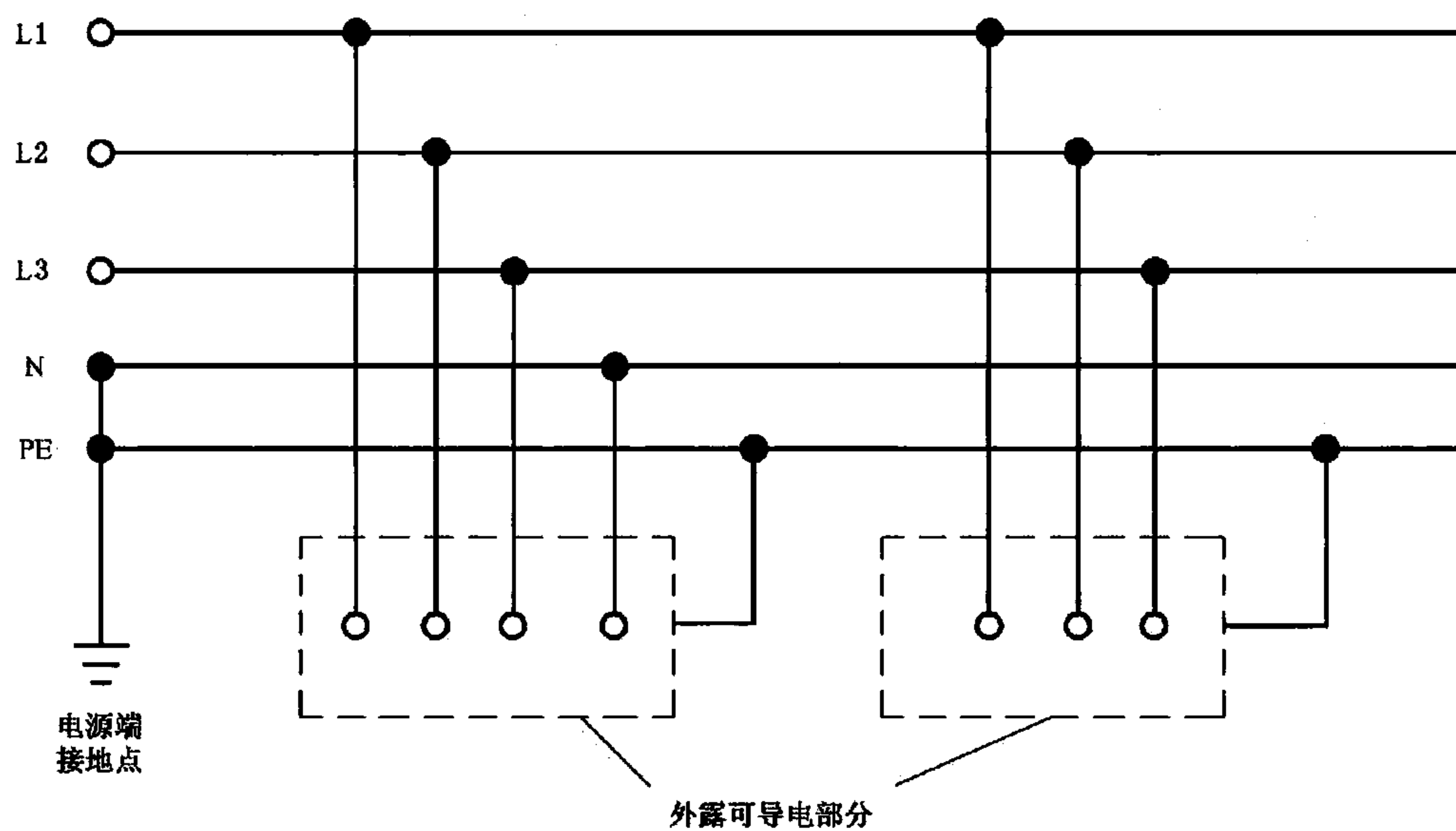
图 1 TN-S 系统
