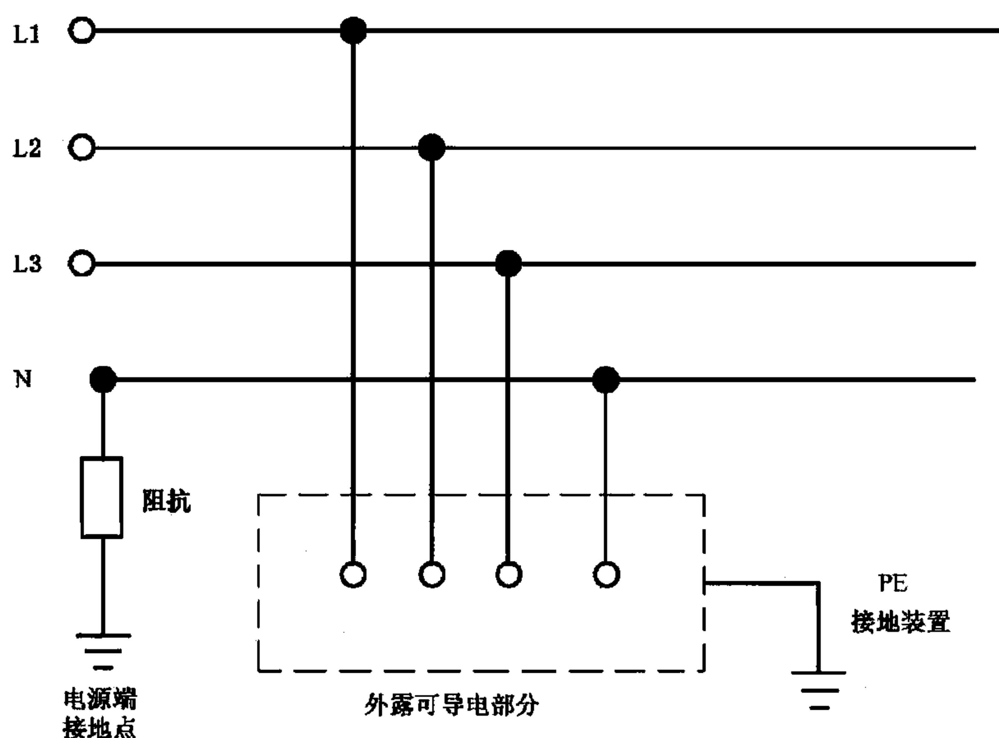
图 5 IT 系统
