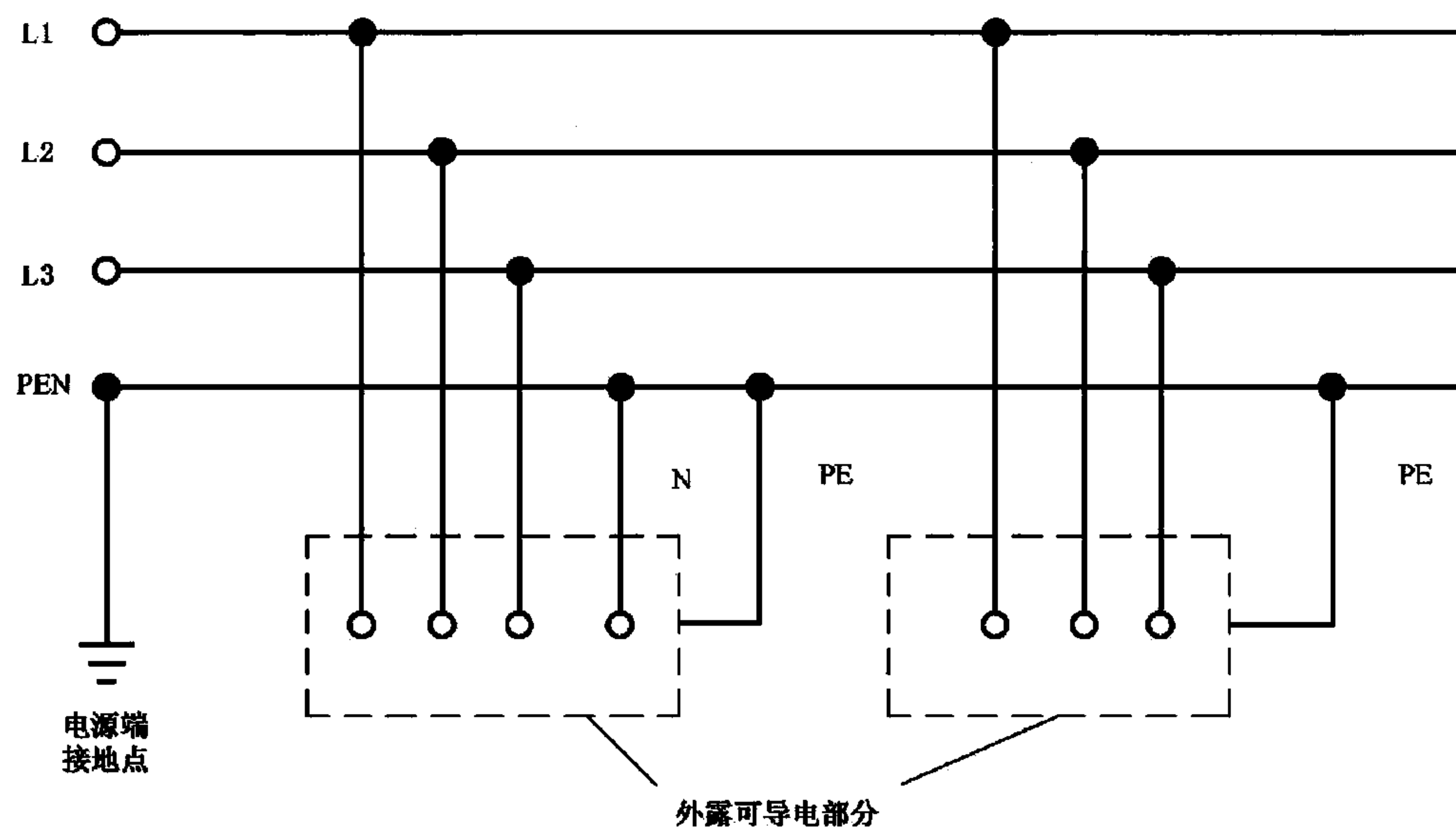
图 2 TN-C 系统
