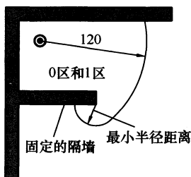
(d) 淋浴间俯视图(有固定隔墙和围绕隔墙的最小半径距离)
