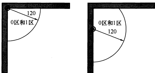
(c) 淋浴头安装在不同位置的俯视图
