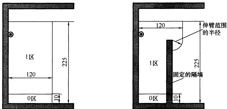
(a) 淋浴间侧视图
