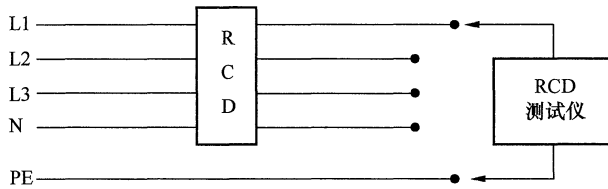
图 1 测试方法
