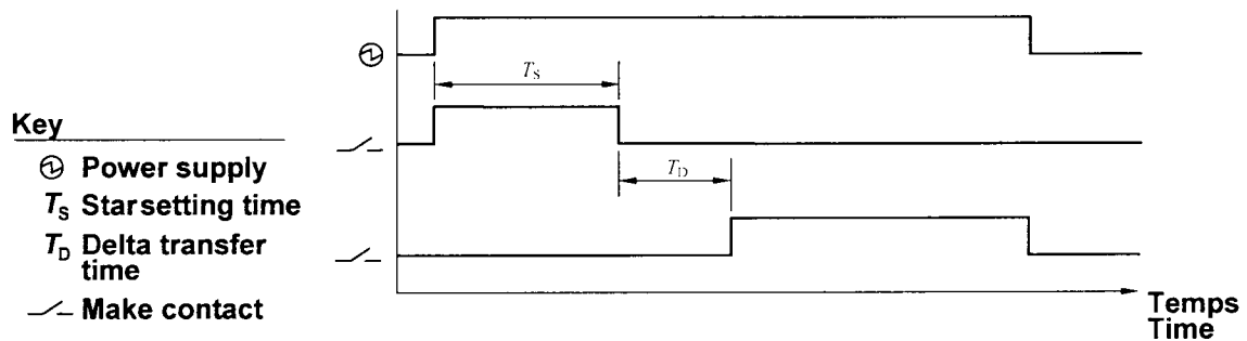
图6 星-三角继电器
