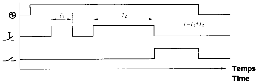
图7 累加时间继电器
