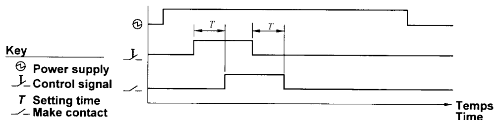
图 4 有控制信号的动作和释放延时继电器
