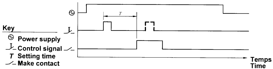
图 9 有控制信号的脉冲延时继电器
