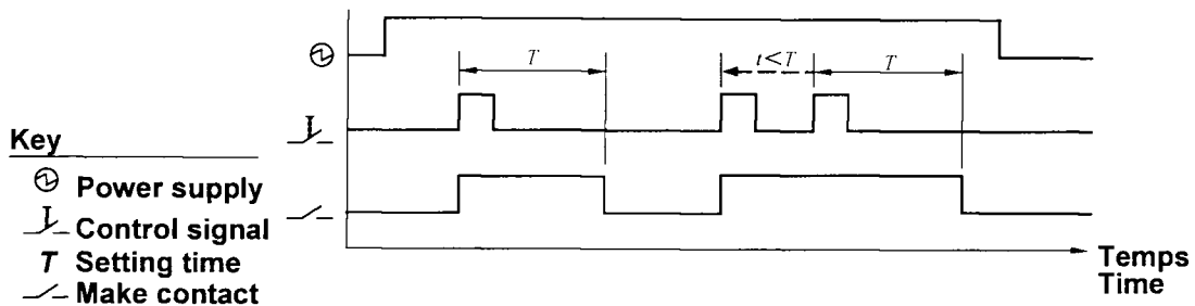
图 12 控制信号接通时重新启动的间隔定时继电器
