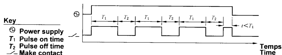
图 5 闪光继电器
