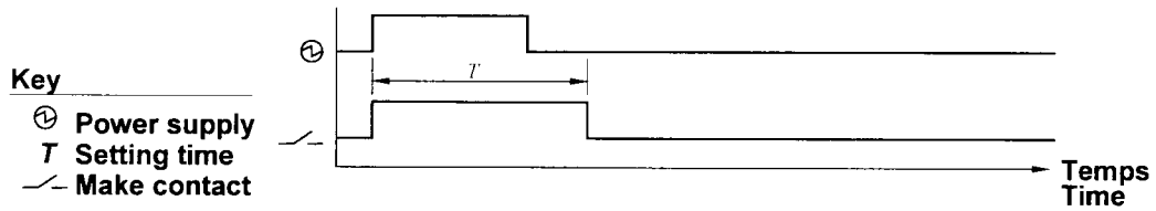
图 14 保持式时间继电器
