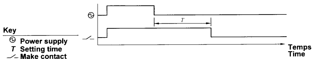
图 2 释放延时继电器
