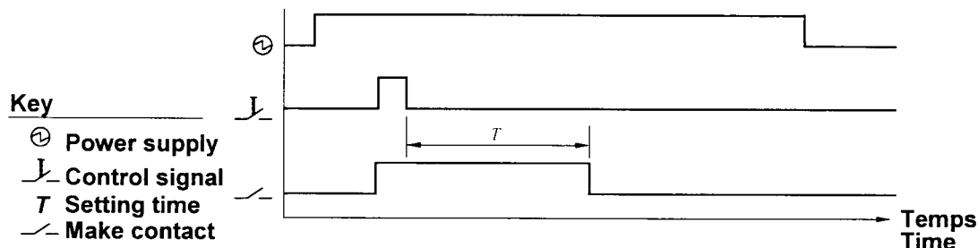
图 3 有控制信号的释放延时继电器
