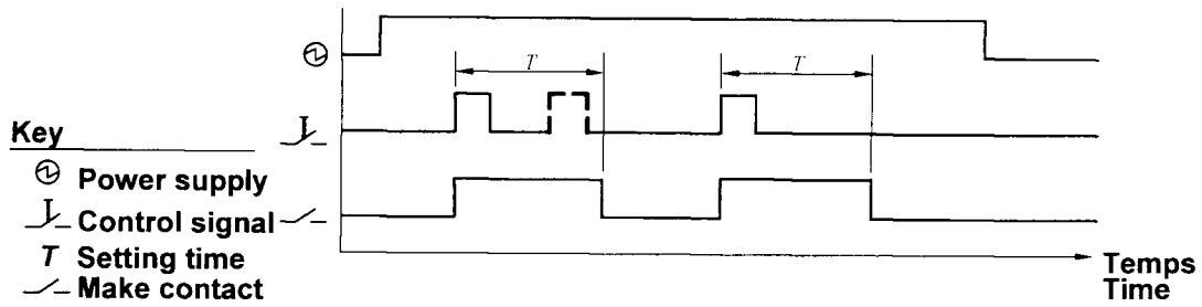
图 11 有控制信号的间隔定时继电器
