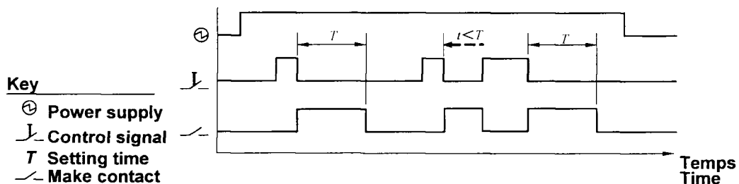
图 13 控制信号关断时重新启动的间隔定时继电器
