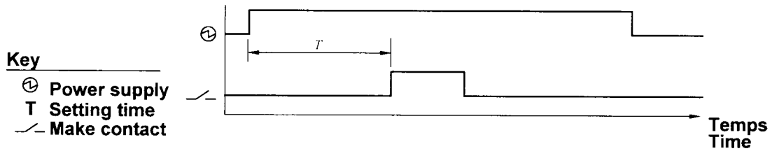
图 8 脉冲延时继电器
