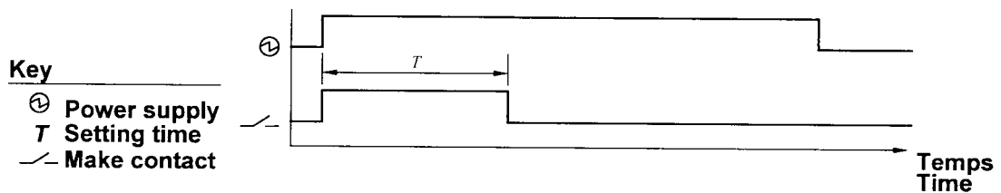
图 10 间隔定时继电器
