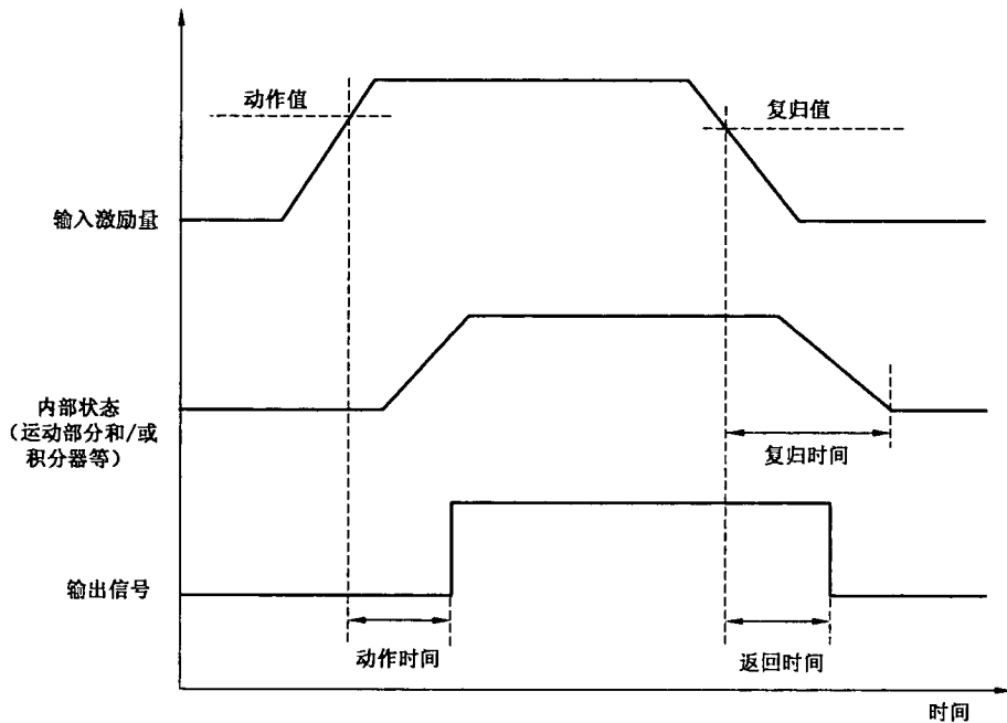
图 1 动作时间、返回时间和复归时间的说明图
