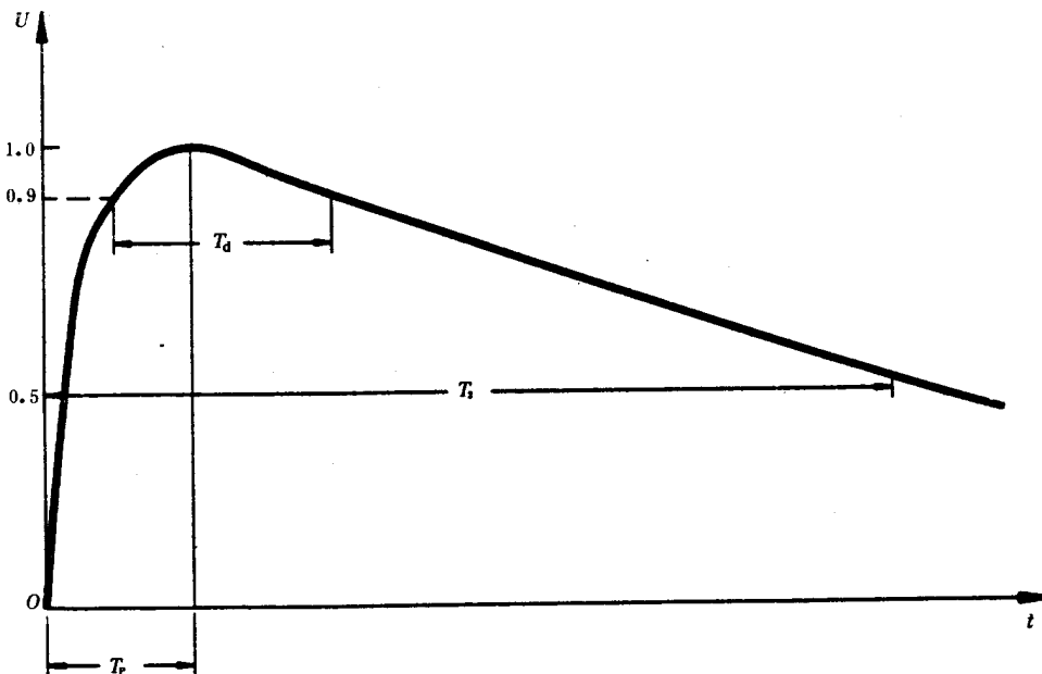
图 7 操作冲击
