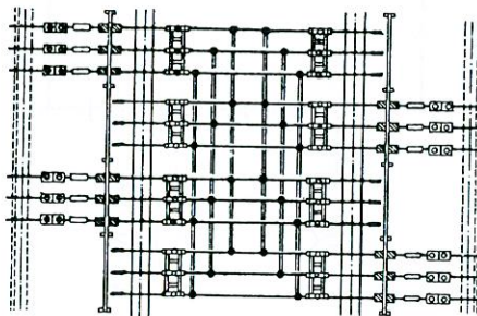
图4 变电路布置
