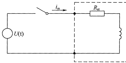
图 2 基本电路
