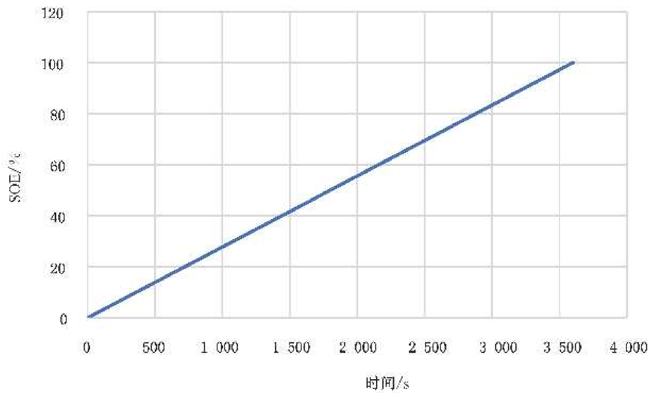
图 D.2 电池充电 SOE-时间曲线
