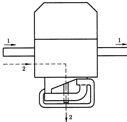
图 5 热短时耐受电流试验布置图
