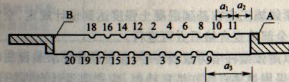
(a) LGJ-95/20钢芯铝绞线
