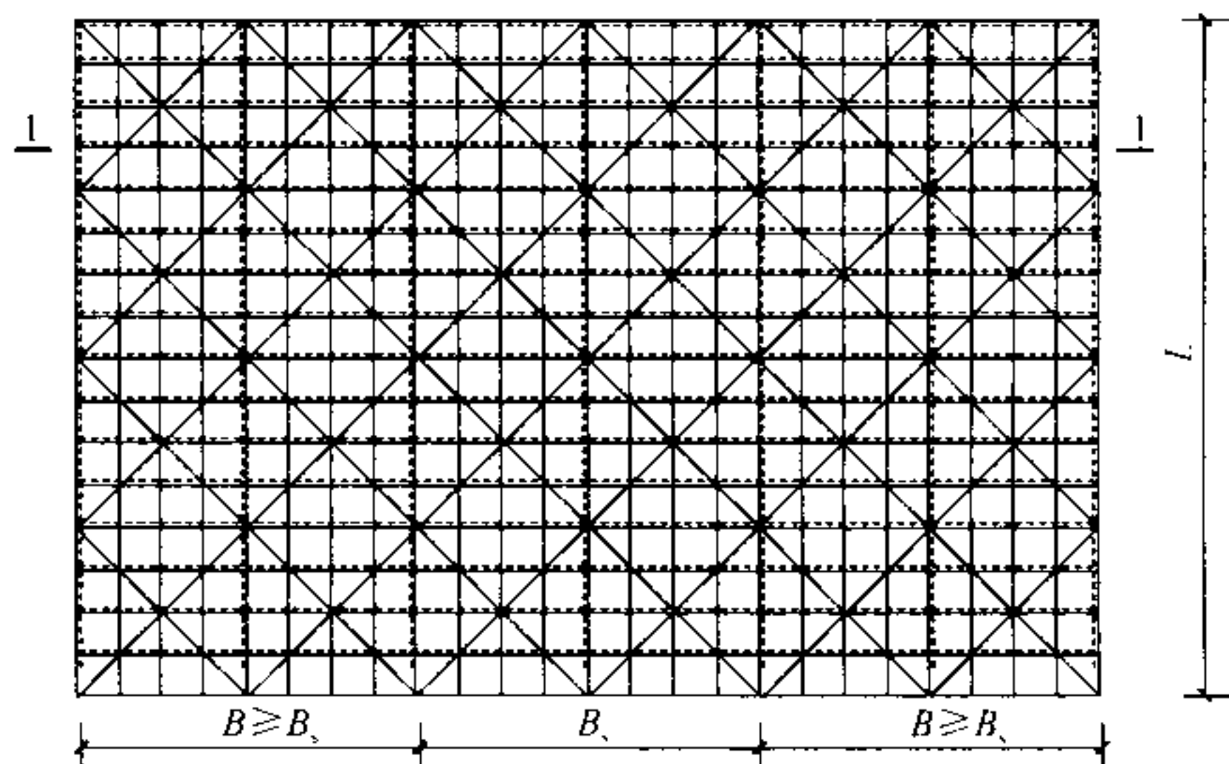
(b) 平面图
