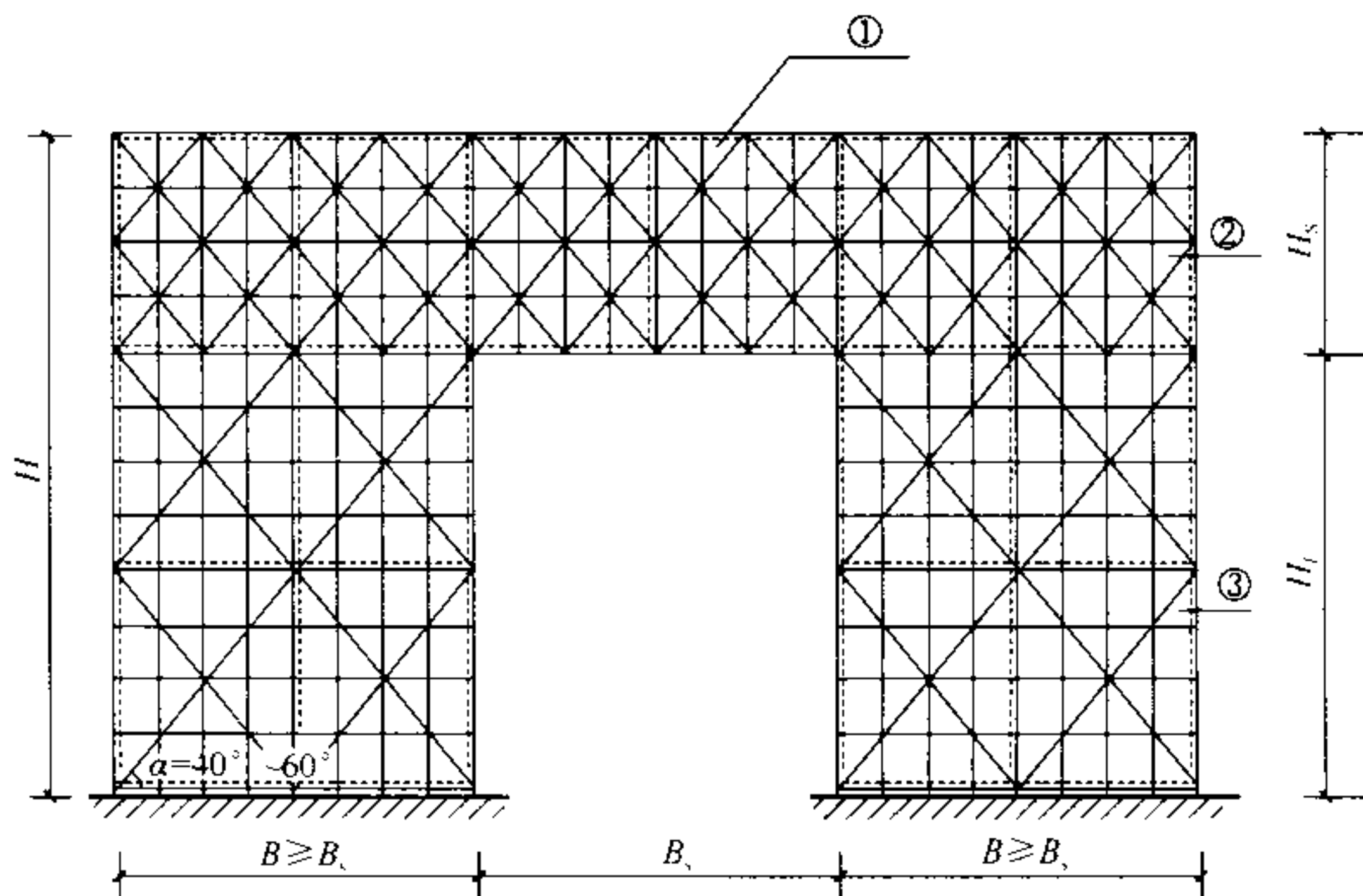
(a) 立面图
