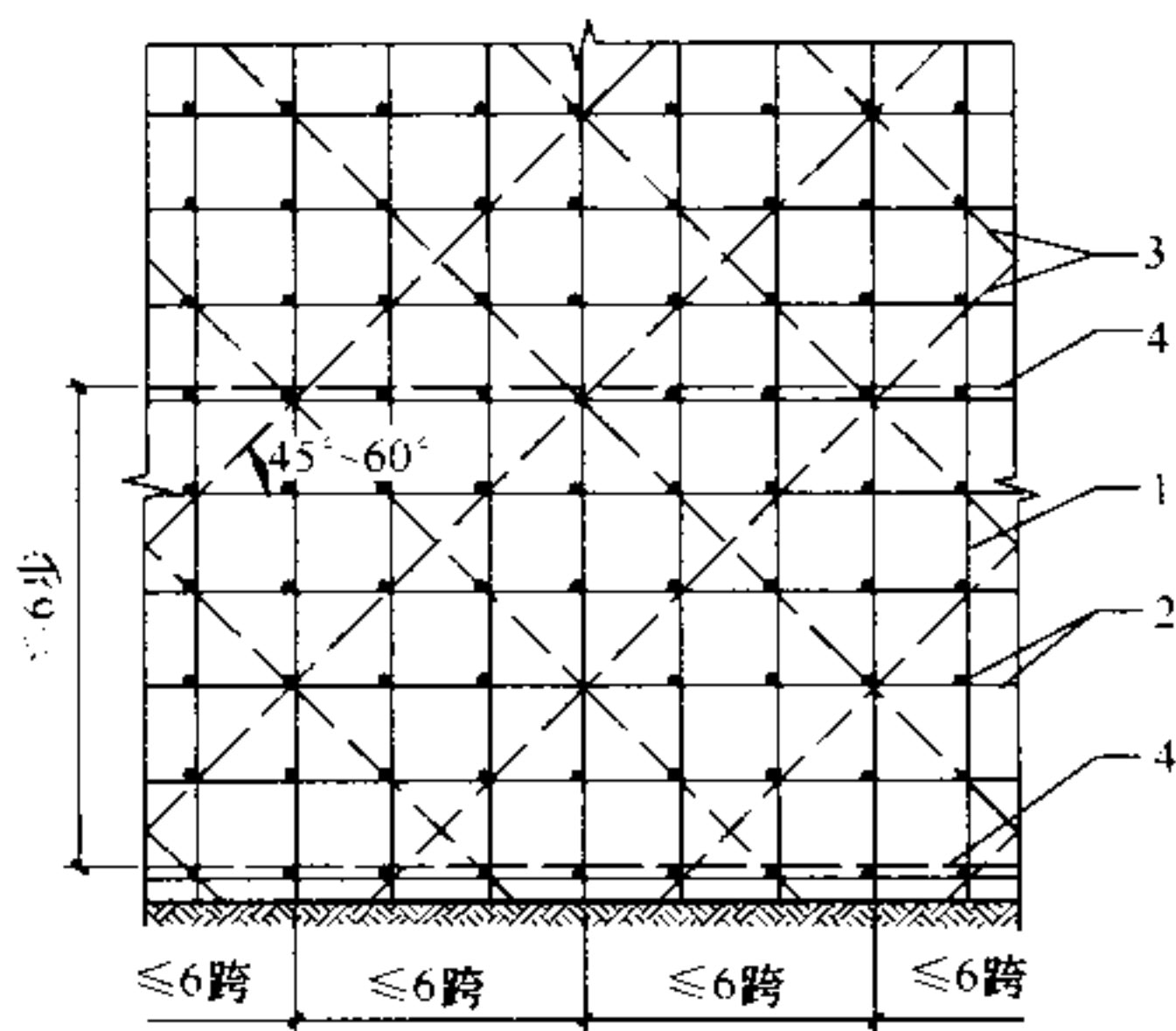
(b) 立面图
