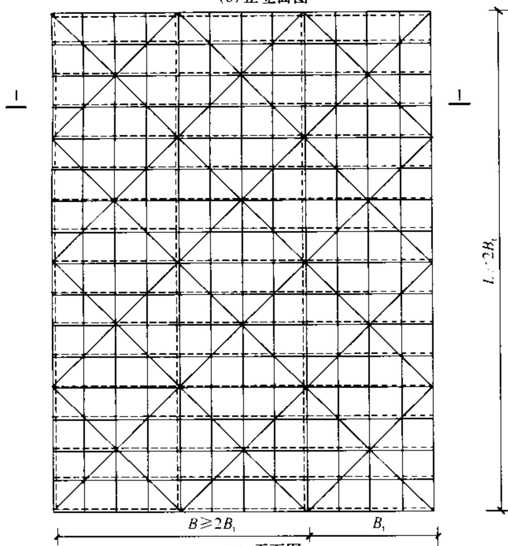
(c) 平面图
