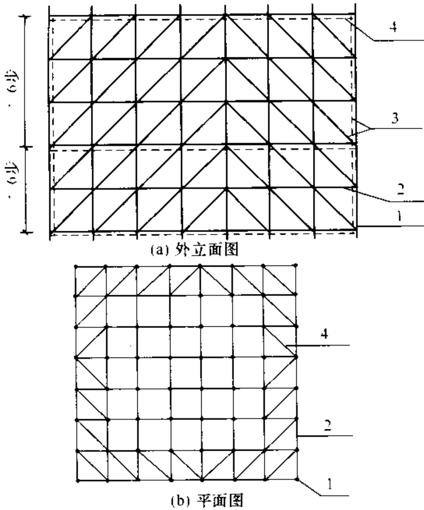
图 5.3.3 桁架式支撑结构斜杆布置图
