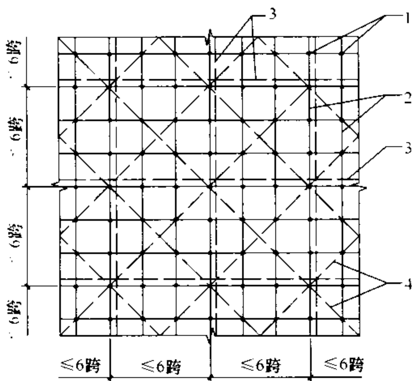
(a) 平面图
