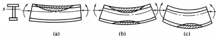
图 1 单轴对称压弯构件失稳时可能的塑性区分布
