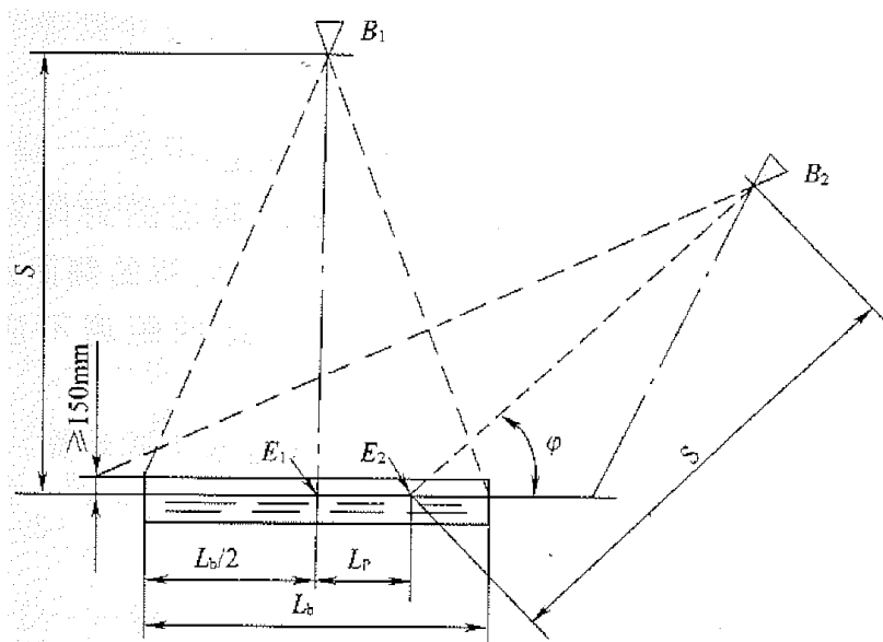
图 3.3.3 架空型喷头布置方法
