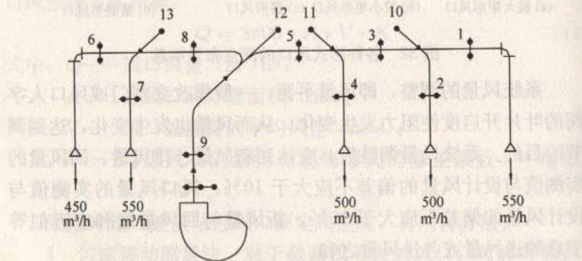
图 34 送风系统
