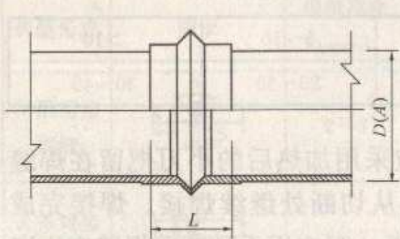
图 5.5.7-1 伸缩节示意
