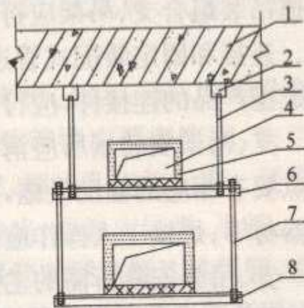
图 23 垂直布置双风管吊架示意
