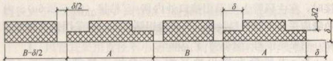
图 5.3.2-1 玻璃纤维复合风管 90°梯形槽口示意 \delta —风管板厚；A—风管长边尺寸；B—风管短边尺寸
