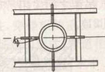
图 16 穿楼板管道 固定支架示意
