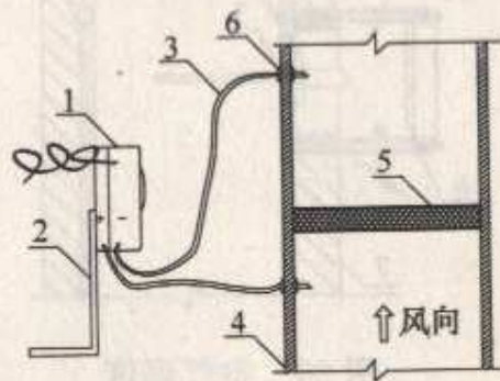
图 27 空气压差传感器（压差开关）安装示意
