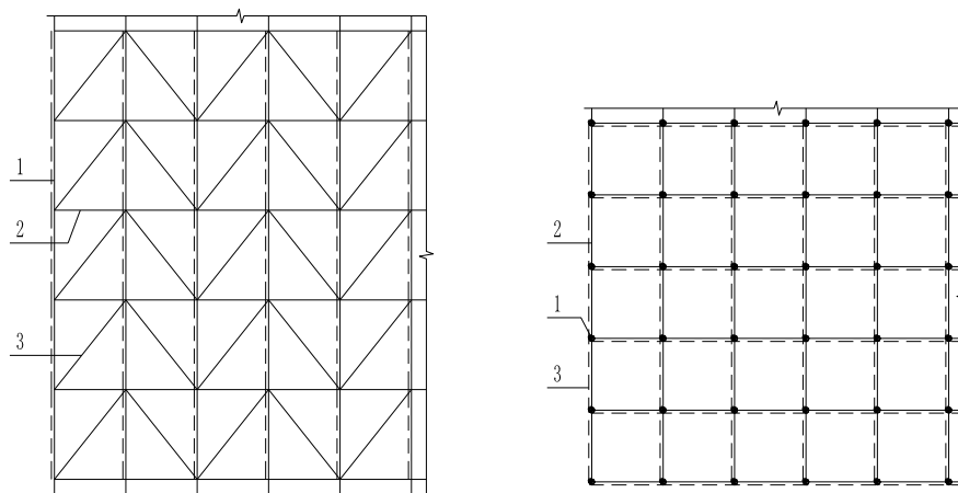
(a) 立面图
