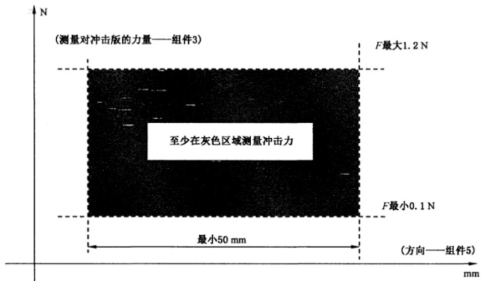
图 11 冲击力分布
