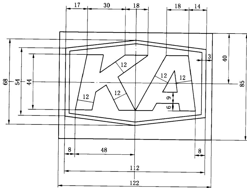
图 4 金属非金属矿山矿用产品安全标志标识图形及参数
