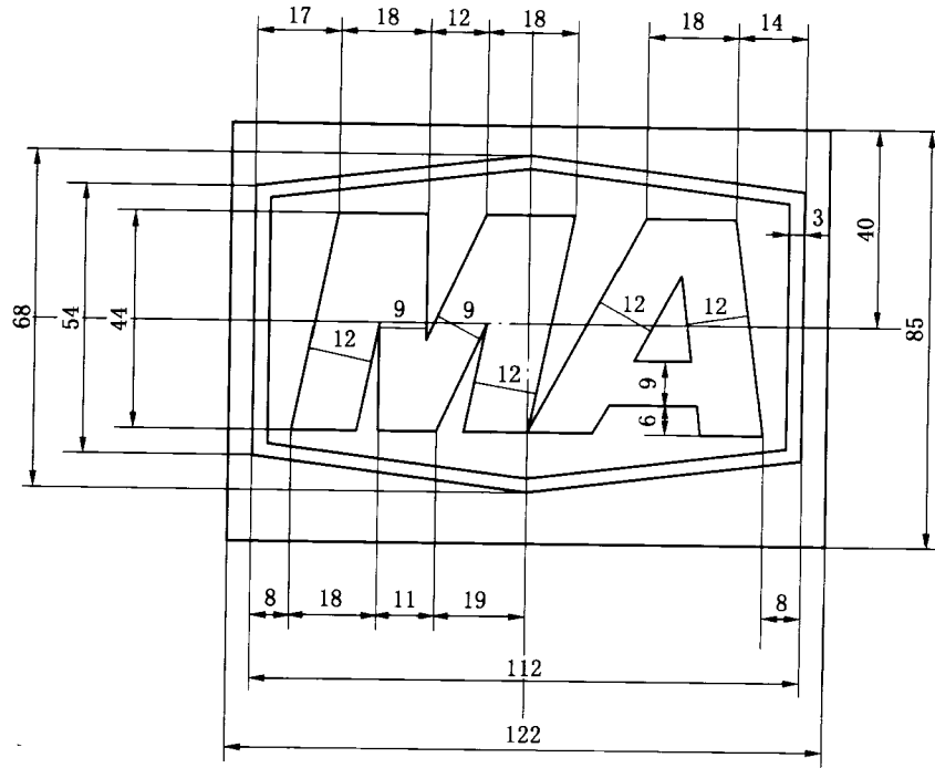
图 3 煤矿矿用产品安全标志标识图形及参数
