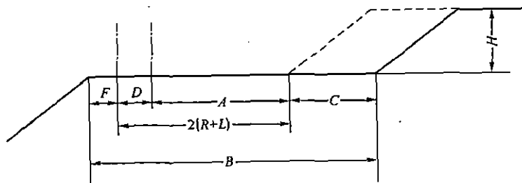
图1 排土场工作平台宽度
