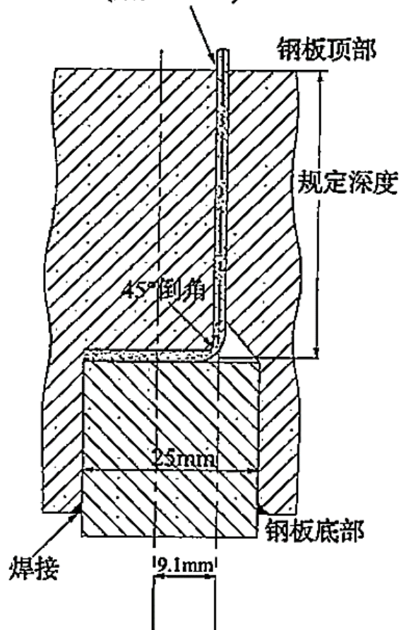
图 A.2.11-2 喷雾冷却试验热电偶布置
