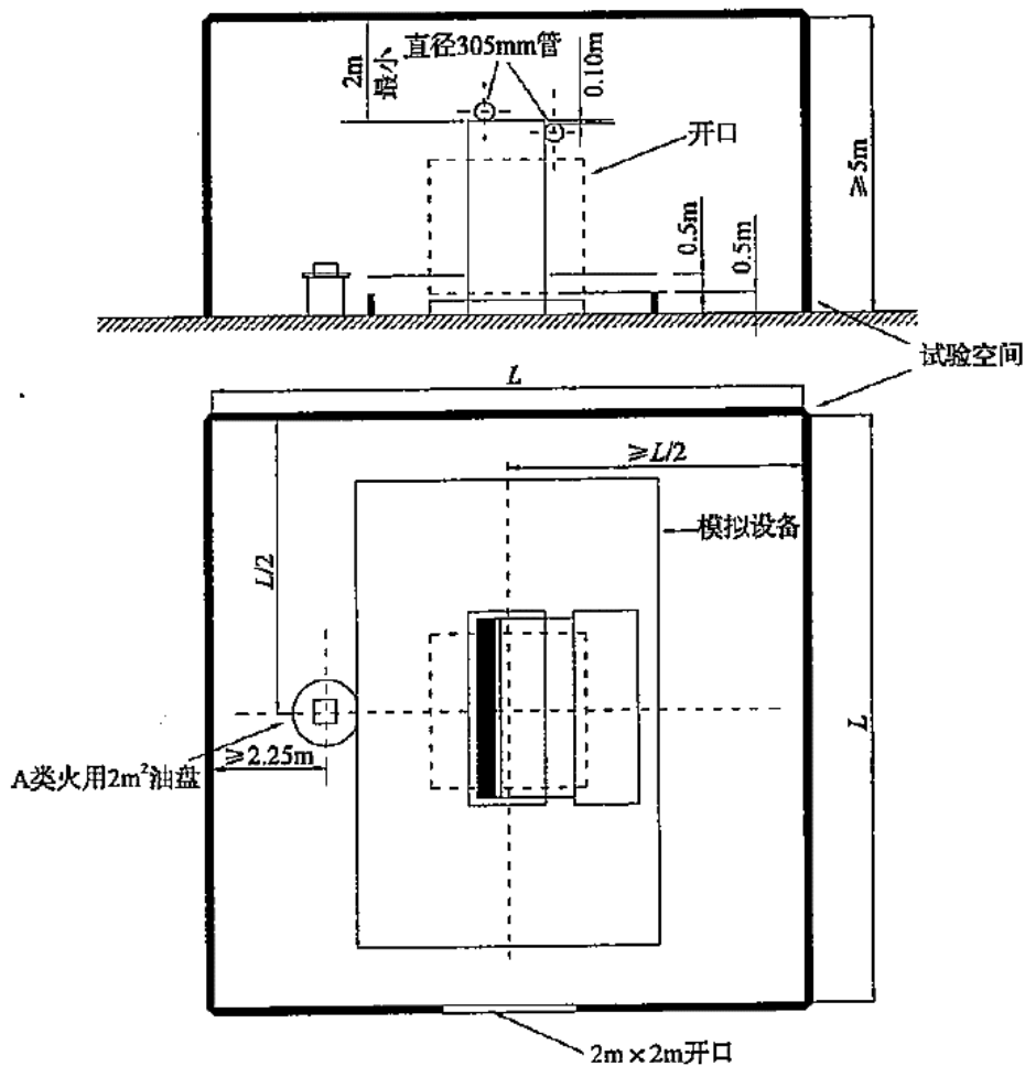
图 A.3.2-1 试验空间和设备模型
