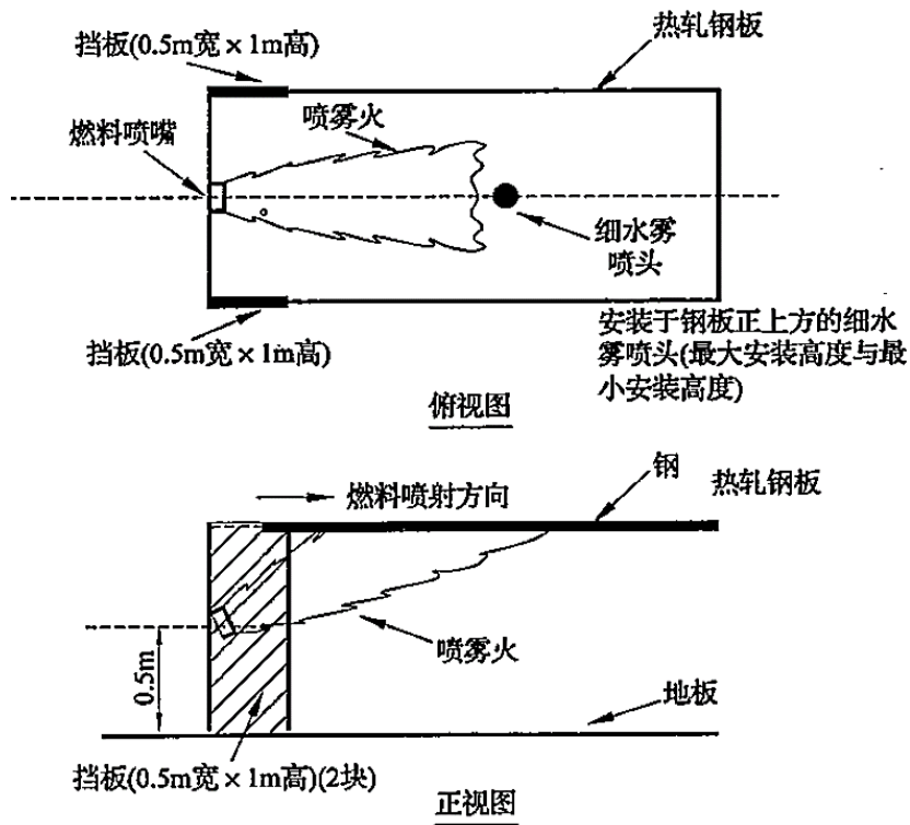
图 A.2.11-1 喷雾冷却试验布置 用于放置热电偶 (直径1.6mm)
