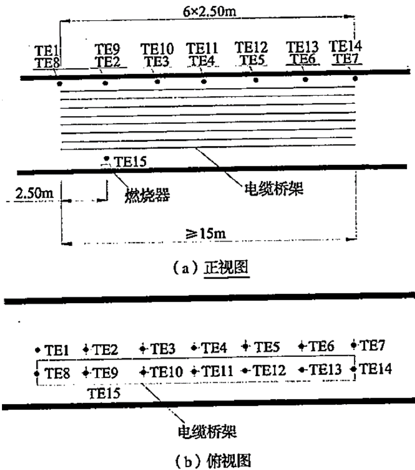
图 A.4.4 试验热电偶布置
