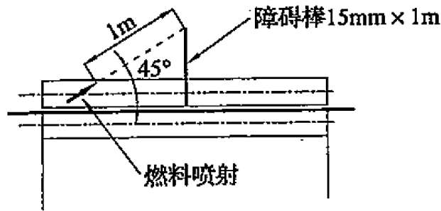
图 A.3.4 倾斜喷雾火的喷嘴布置位置
