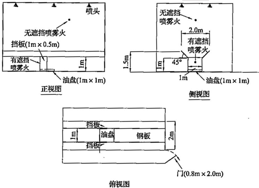
图 A.2.2 试验空间和设备模型
