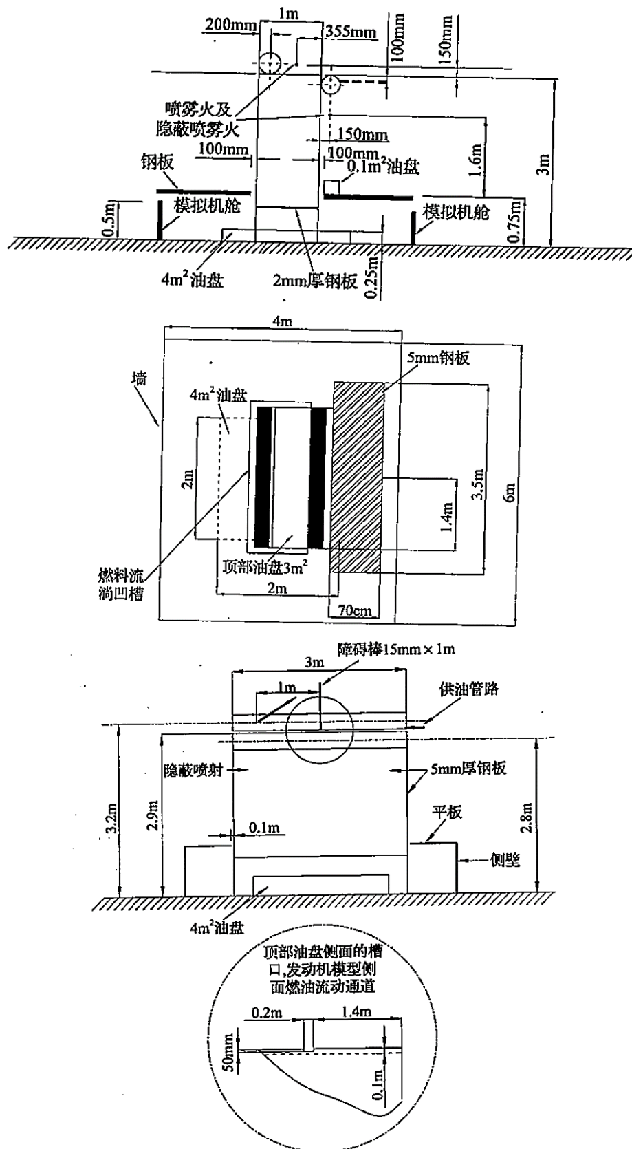
图 A.3.2-2 设备模型和试验设施布置
