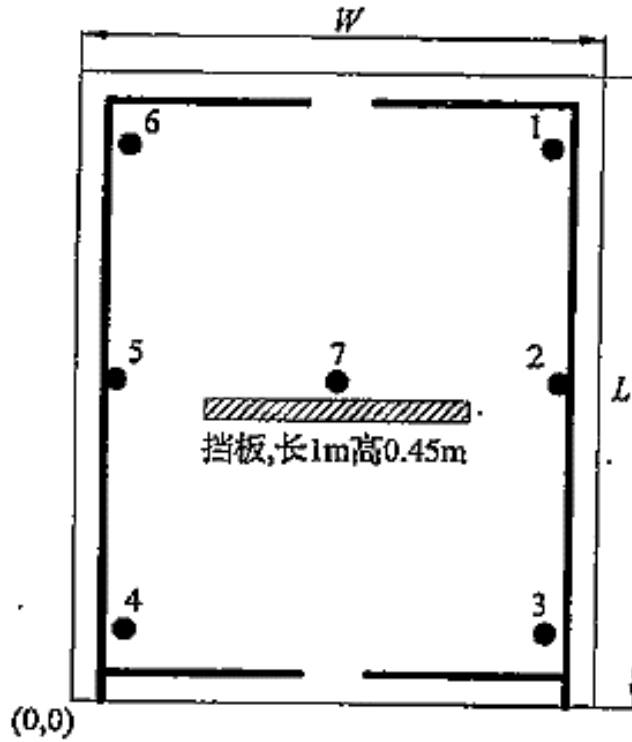
图 A.5.2-1 油罐火位置
