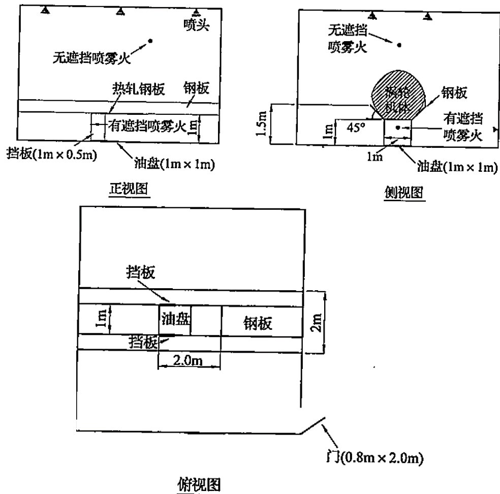
图 A.2.9 试验空间和涡轮机模型
