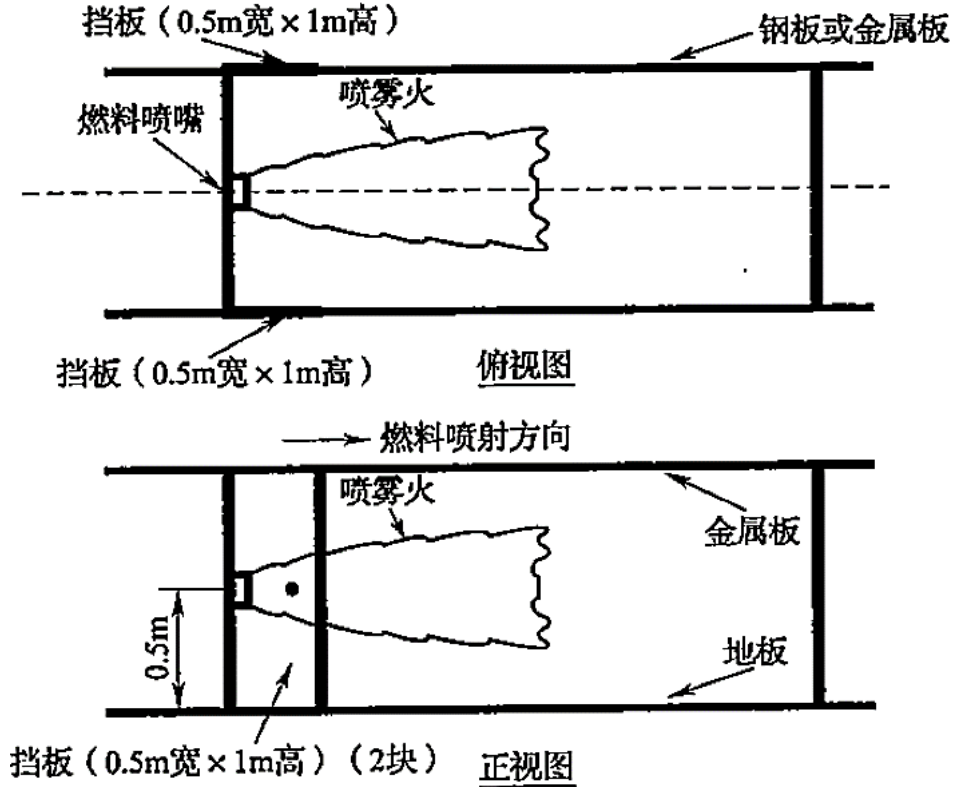
图 A.2.4-1 火源和遮挡喷雾火布置
