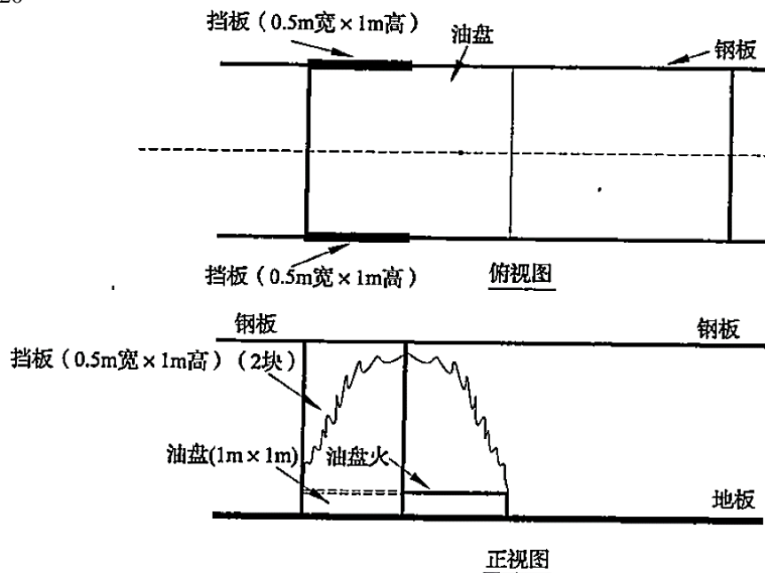
图 A.2.4-2 火源和遮挡油盘火布置
