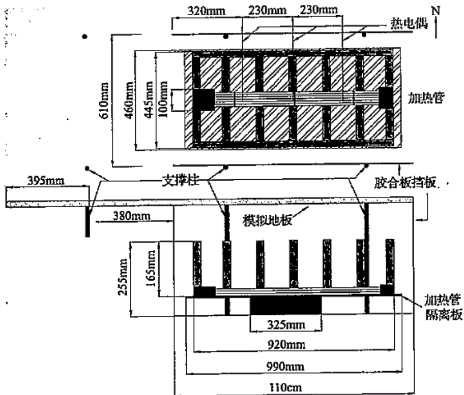
图 A.5.2-2 电缆火燃烧物示意
