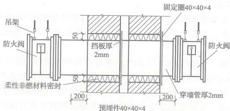
图 9 变形缝处的防火阀
