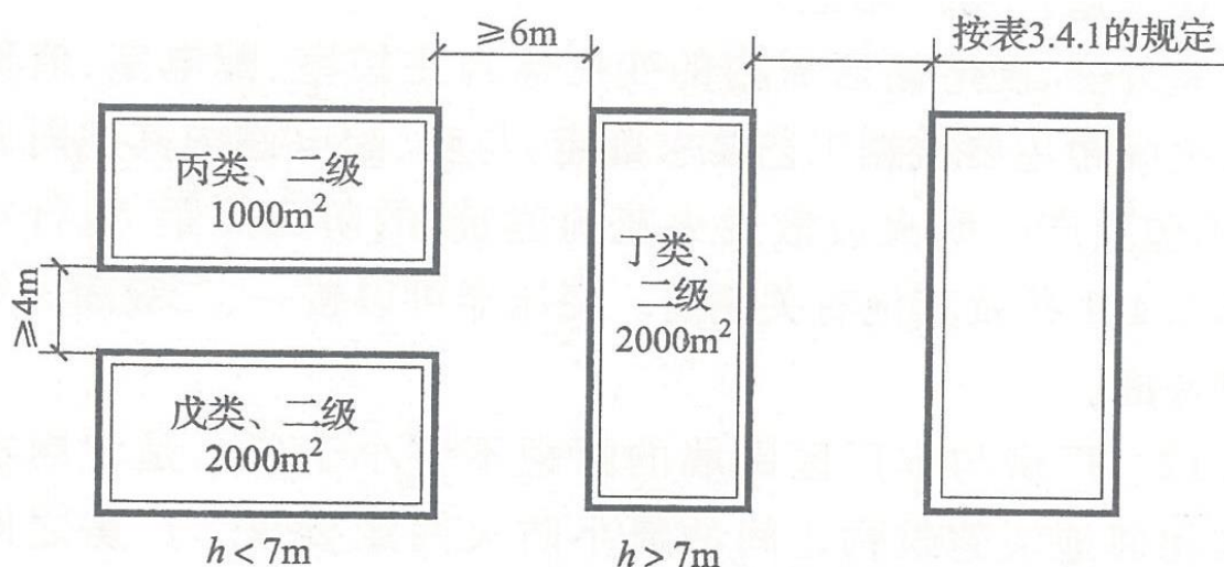
图4 成组厂房布置示意图
