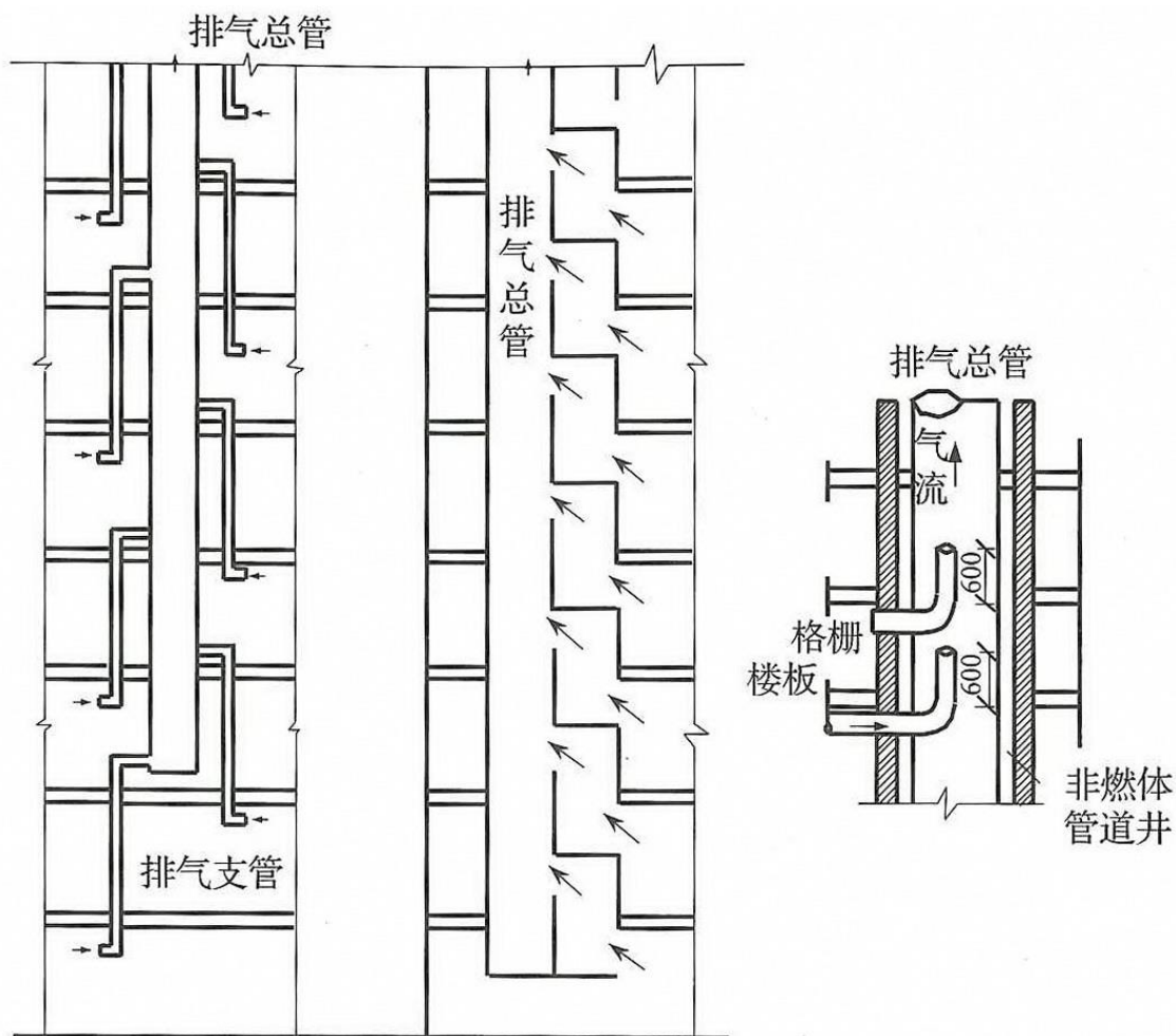
图 8 排气管防止回流示意图
