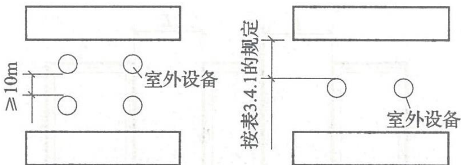
图 1 有室外设备时的防火间距
