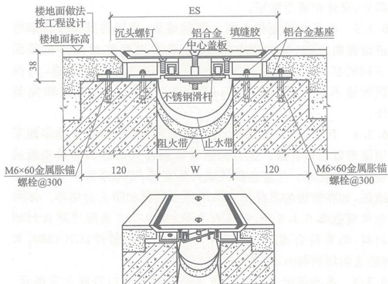
图 7 变形缝构造示意图
