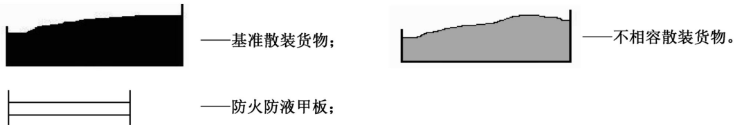
图 2 固体散装危险货物之间隔离示意图
