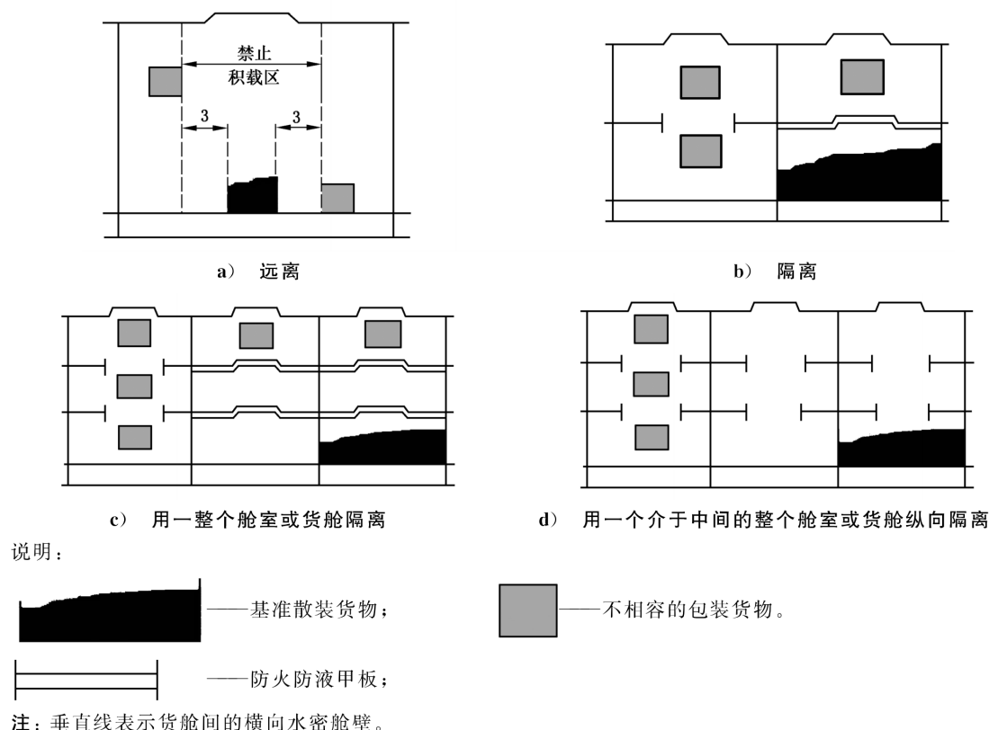
图 1 固体散装危险货物与包装危险货物隔离示意图
