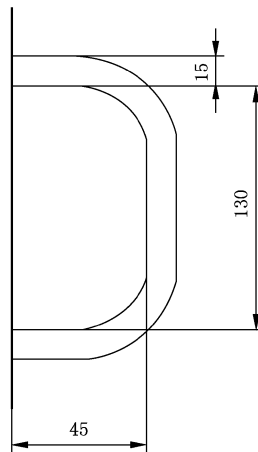
图 3 抓手
