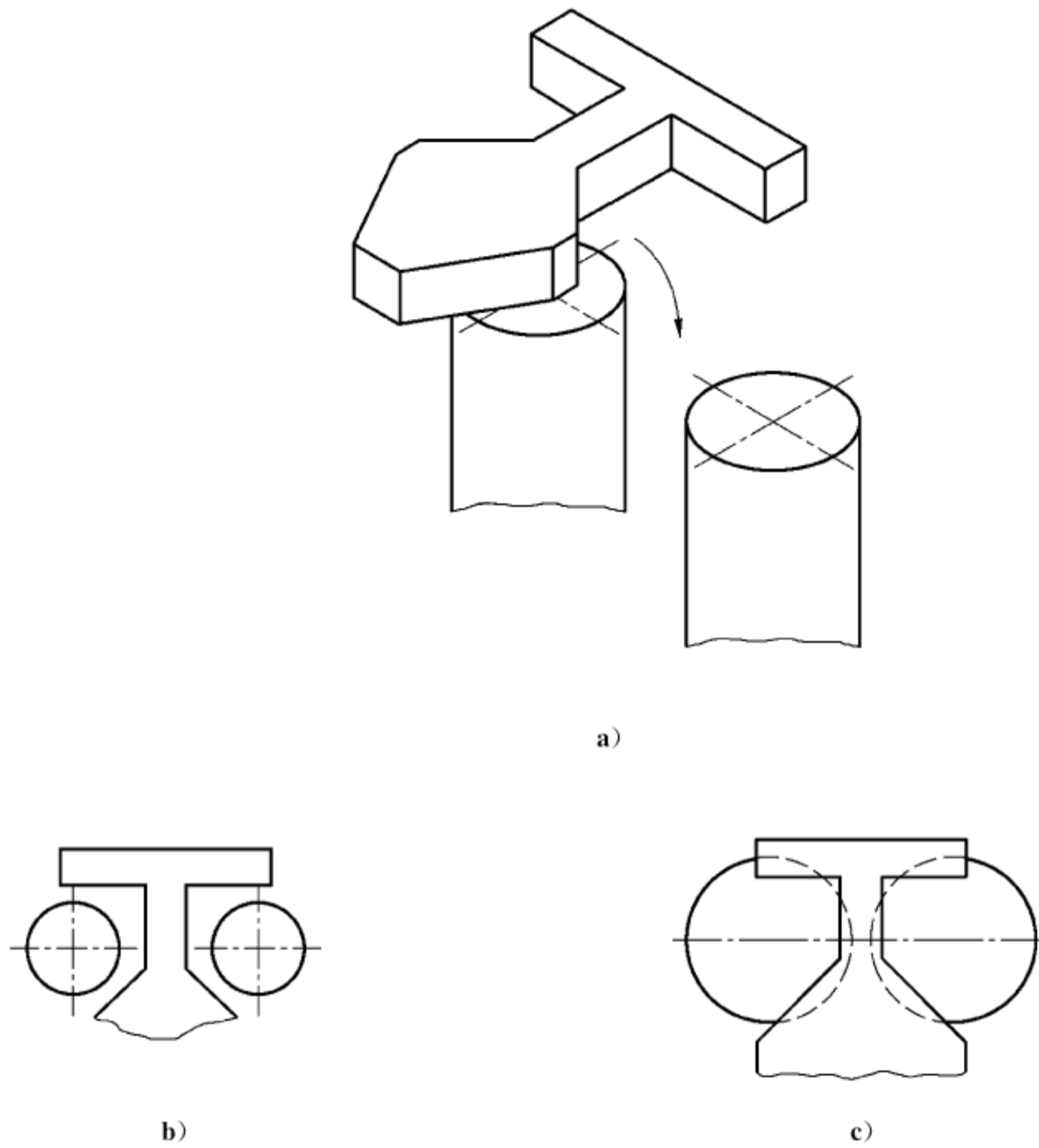
图 C.4 使用测试模板“B”部分的方法
