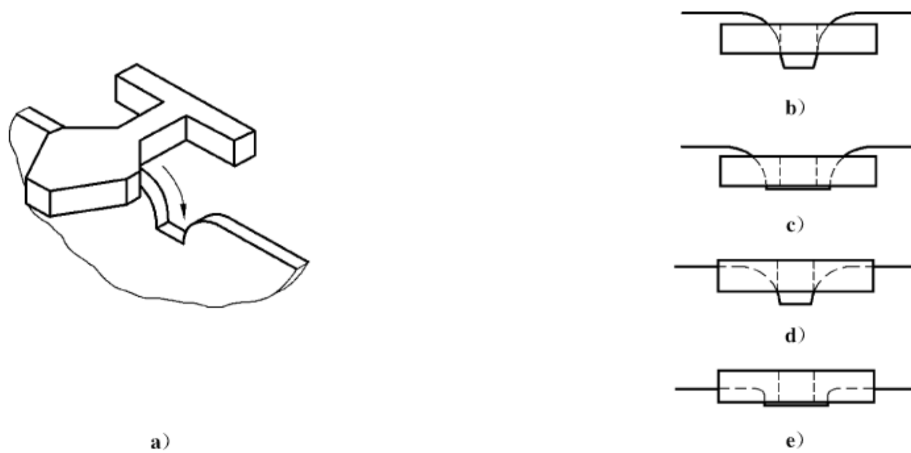
图 C.3 使用测试模板“B”部分的方法
