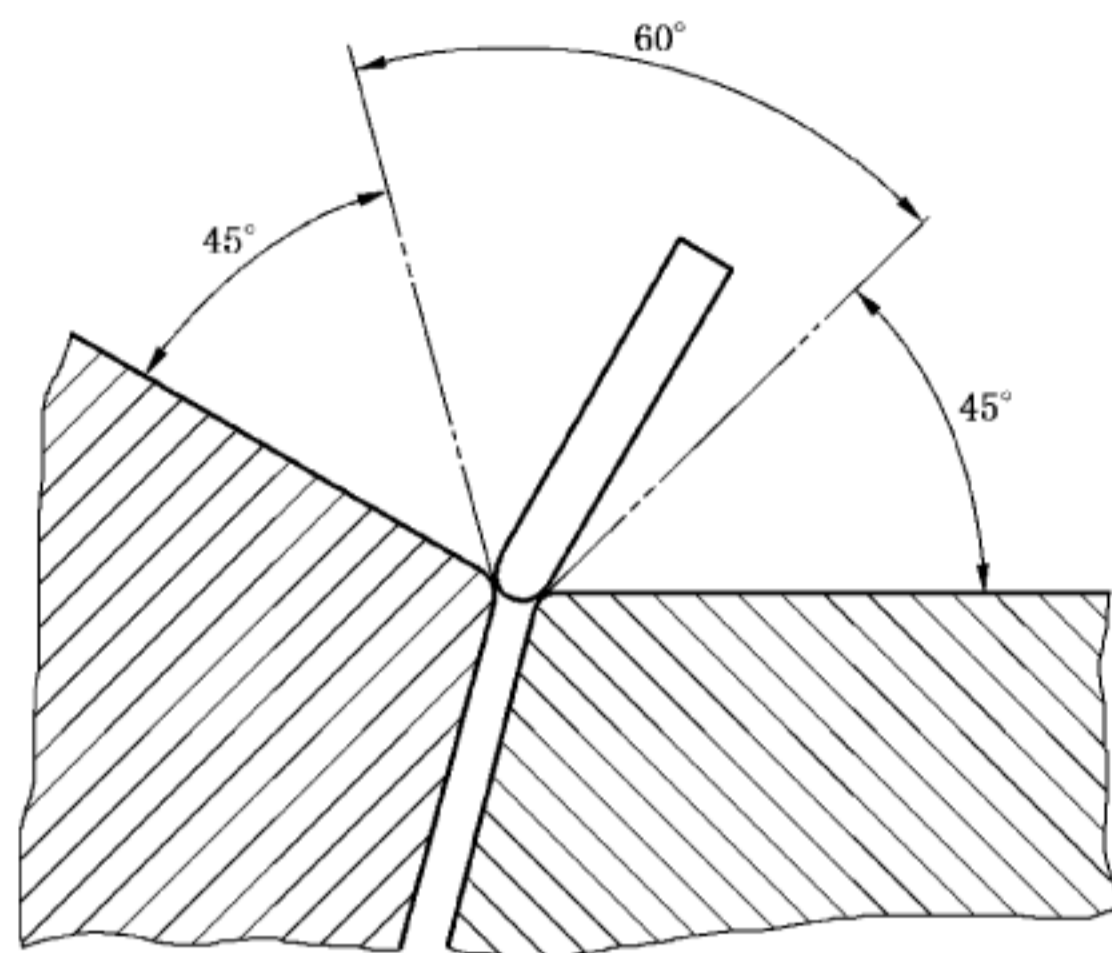
图 C.11 8 mm 测试指转动范围
