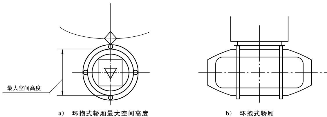
图 C.2 回转式轿厢放大示意图
