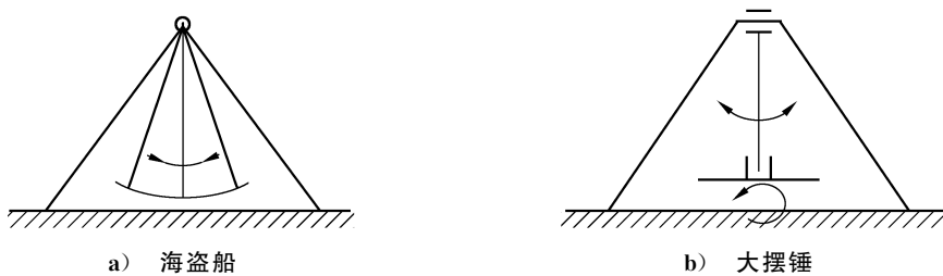
图 A.3 摆锤型(C型)
