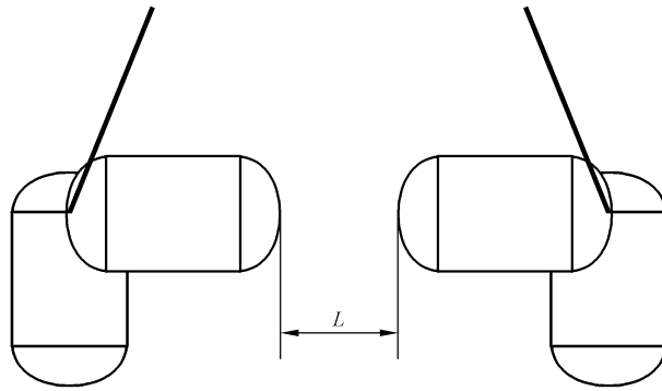
图 C.4 轿厢翻转时需留有距离 L 示意图
