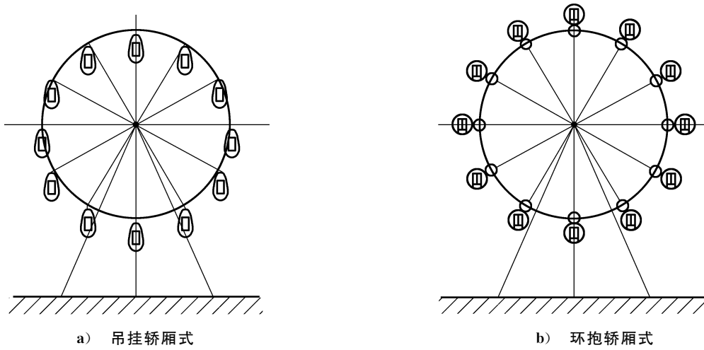
图 A.1 有主轴摩天轮型(A型)
