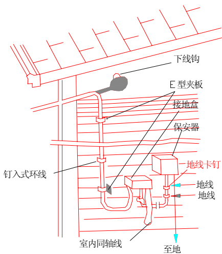
图 3.6.6—1 接地盒
