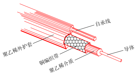
图 3.5.2—1 自承式同轴电缆
