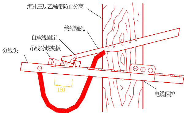
图 3.5.3—1 终结在吊线上
