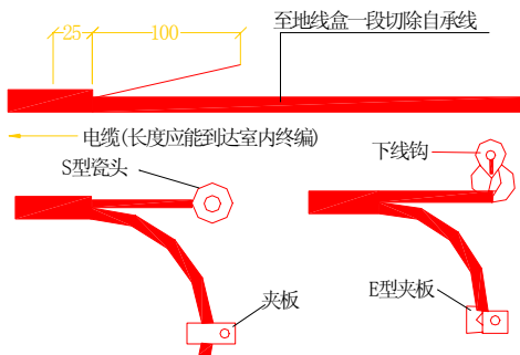
图 3.5.2—2 自承式电缆的自承线
