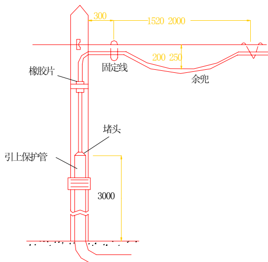
图 3.4.10 地下光缆引出时的保护
