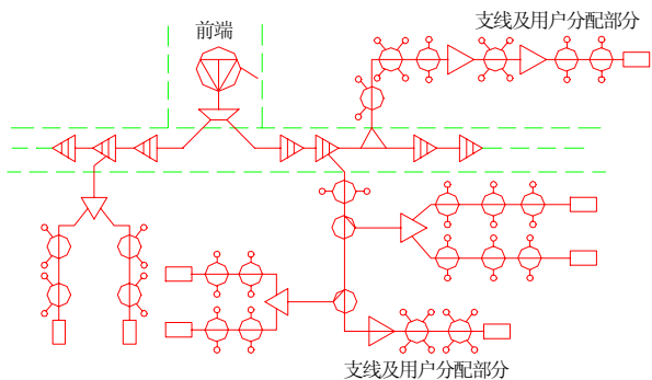
图 2.2.1—2 独立前端系统模式
