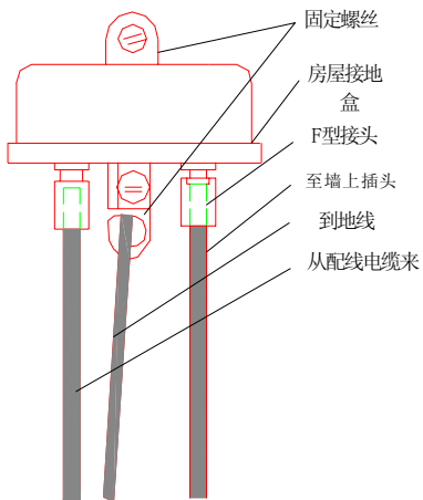
图 3.6.6—1 接地盒
