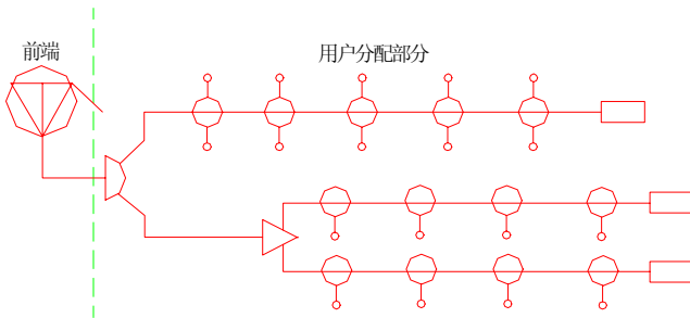
图 2.2.1—1 无干线系统模式
