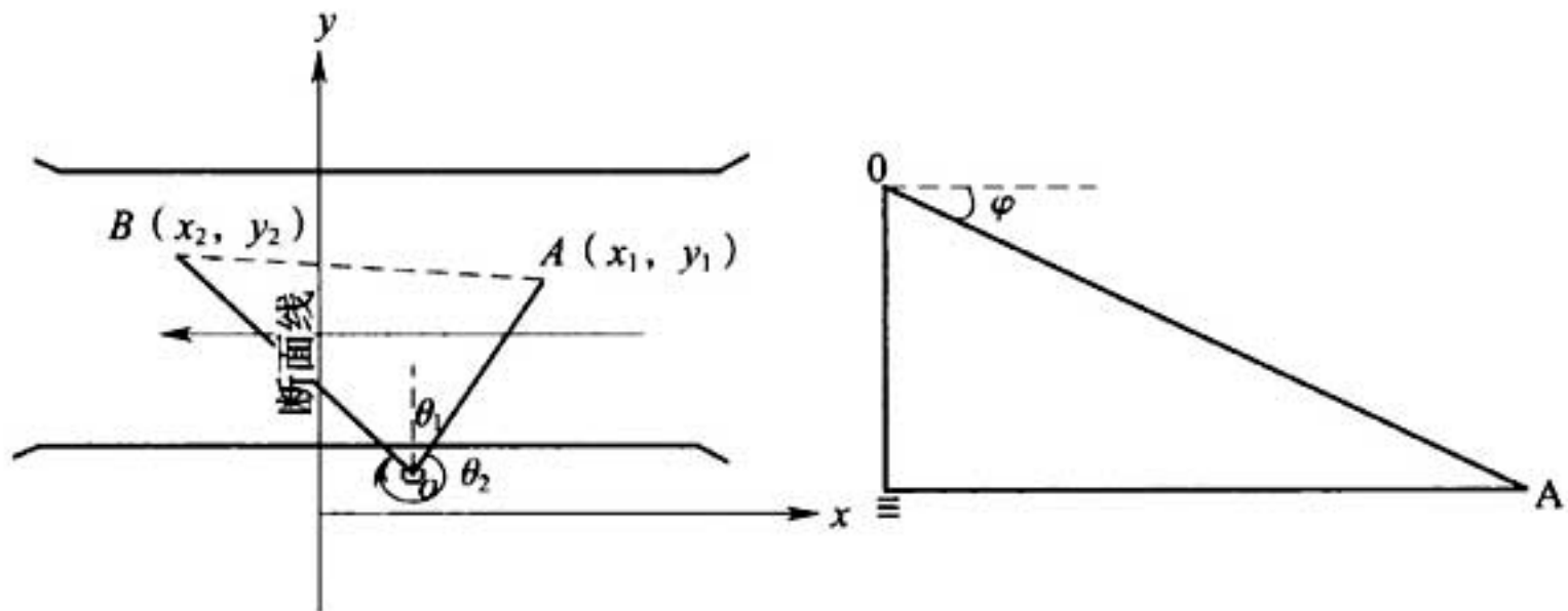
图 C. 7. 7-1 极坐标浮标法测流布置示意图
