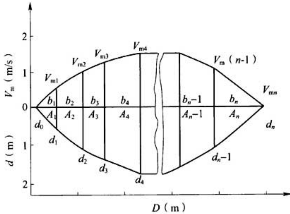
图 B. 7. 1 部分面积计算划分
