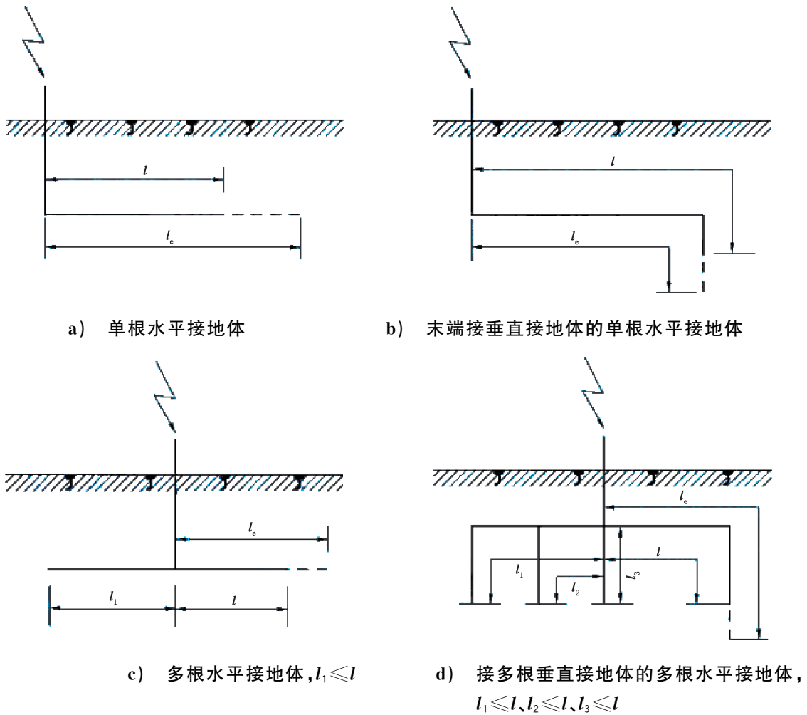
图 A.2 接地体的有效长度的计量
