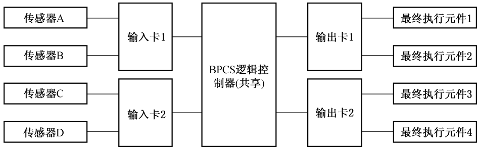
图 D.3 相同场景下共享输入/输出卡的影响
