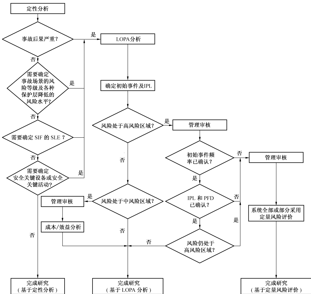
图 B.1 LOPA 的应用时机
