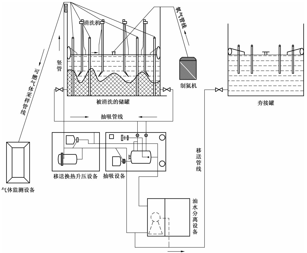
图 A.1 机械清洗工艺流程图
