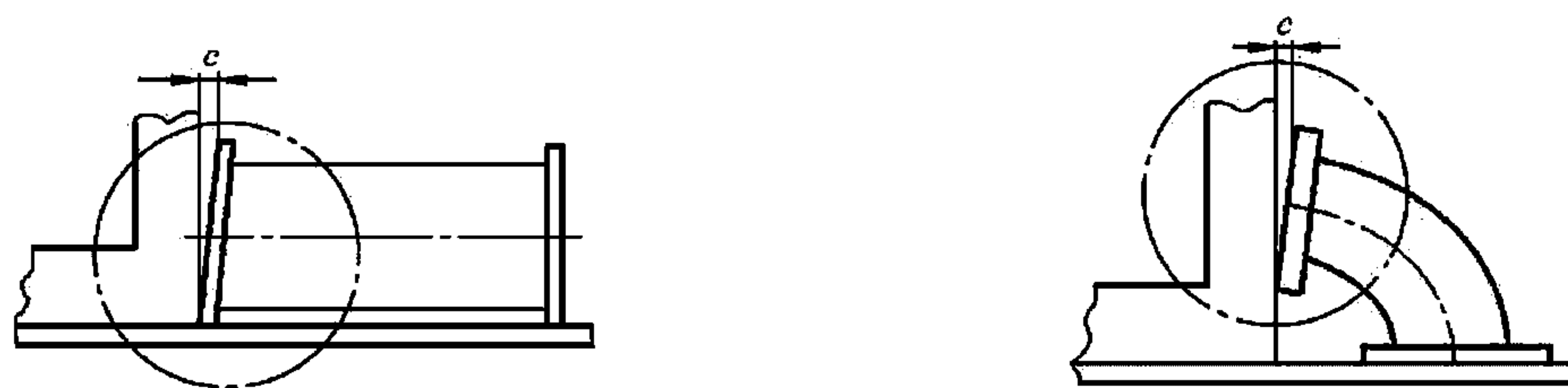
图 1 塔节、管道及管件的形位公差示意图
