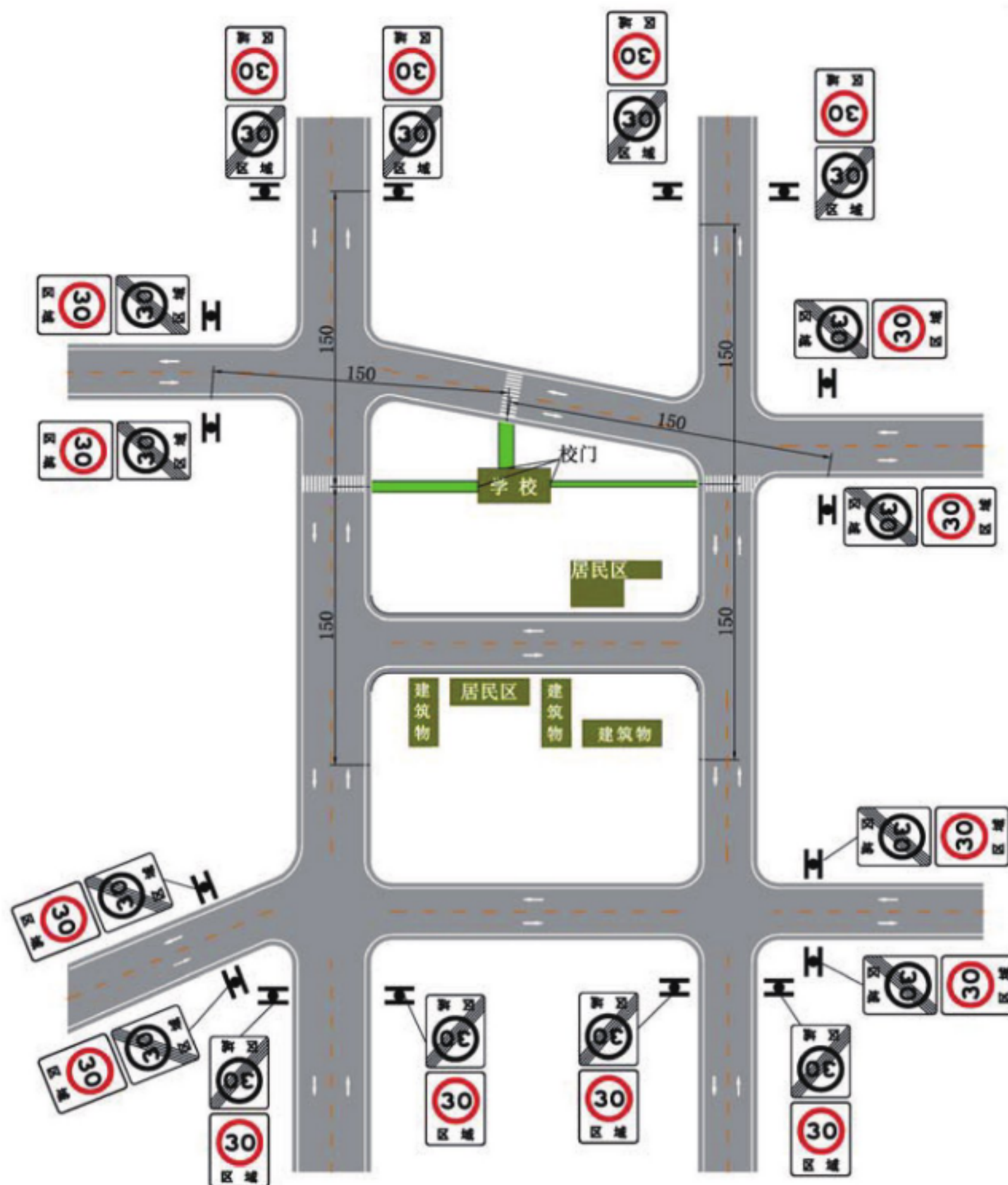
图 2 区域限速标志设置示例
