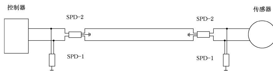
图 B.1 SPD 接线形式图
